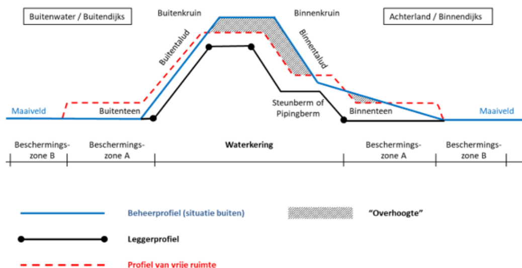
Figuur 20.1: Voorbeeld profiel waterkering met overhoogte
