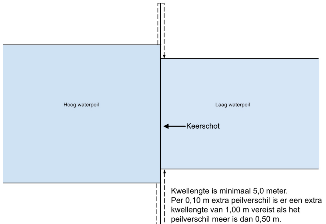
Bovenaanzicht kwellingte langs een keerschot
