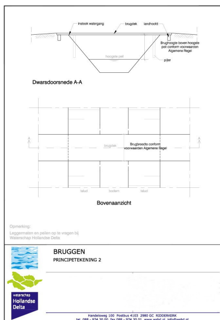
Principetekening 2 Bruggen
