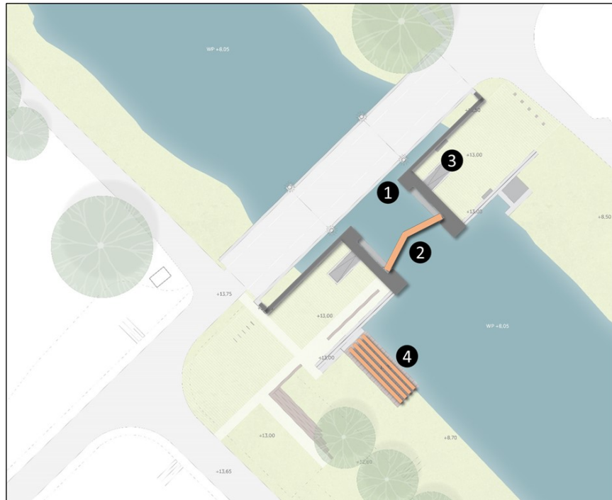
Figuur 3 1: Referentieontwerp Versterking Keersluis Mook
