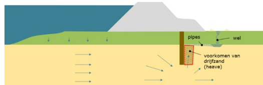
Figuur 4 Werkend principe van een heavescherm
