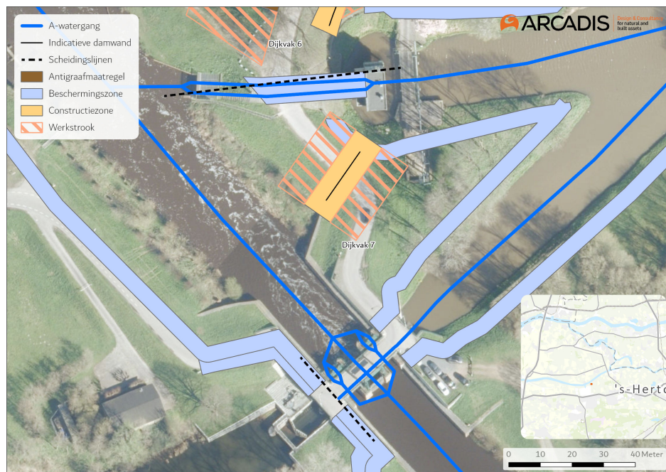
Dijkverbetering Doeveren met (beschermszone) A-watergang dijkvak 7
