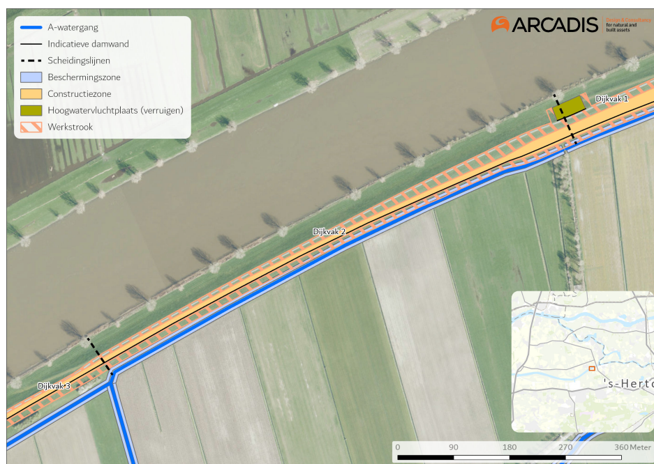
Dijkverbetering Doeveren met (beschermingszone) A-watergang dijkvak 2
