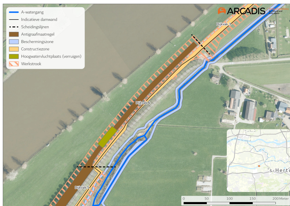
Dijkverbetering Doeveren met (beschermingszone) A-watergang dijkvak 4
