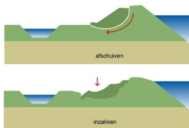
Figuur 2 Schematische weergave macrostabiliteit binnenwaarts
