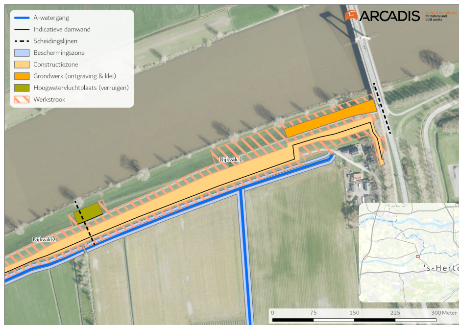
Dijkverbetering Doeveren met (beschermingszone) A-watergang dijkvak 1
