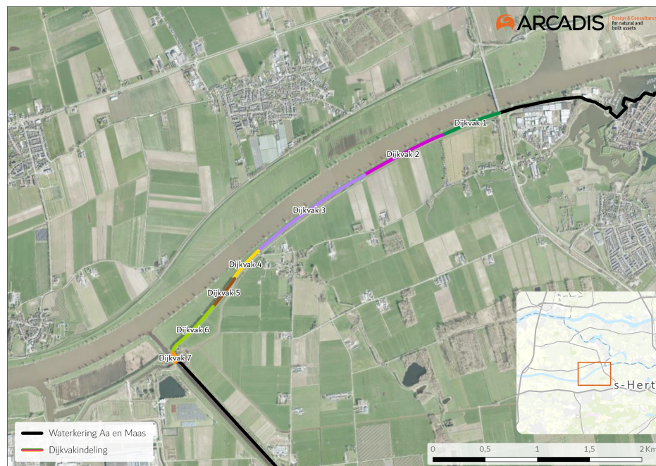
Figuur 7 Overzicht dijktraject en dijkvakken dijkverbetering Doeveren
