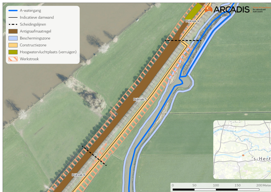
Dijkverbetering Doeveren met (beschermingszone) A-watergang dijkvak 5
