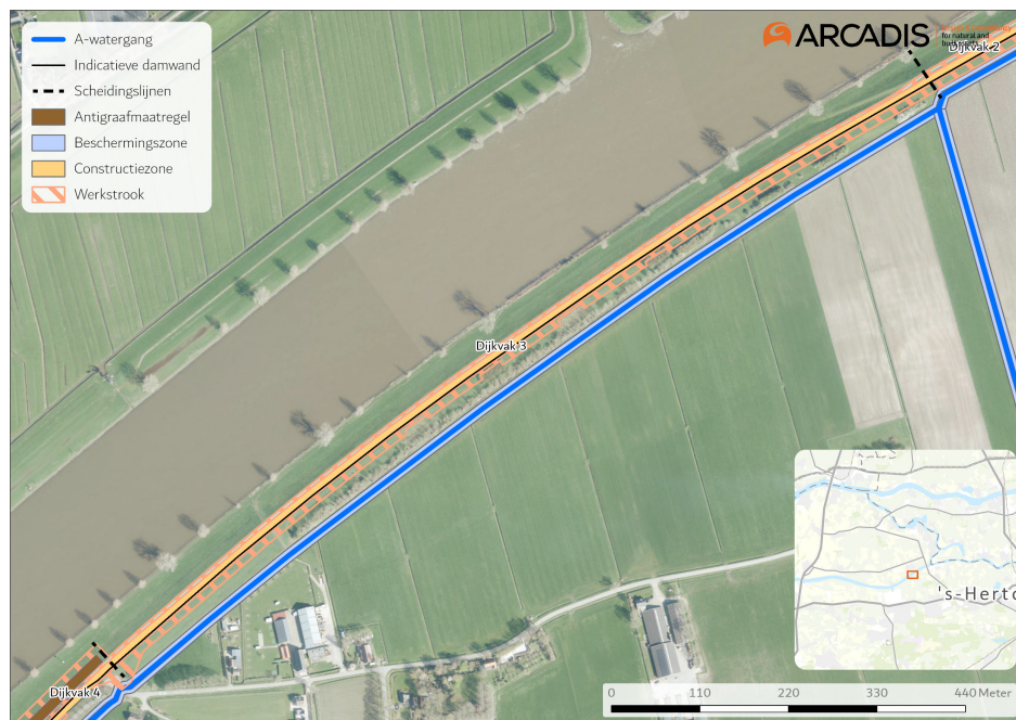
Dijkverbetering Doeveren met (beschermingszone) A-watergang dijkvak 3
