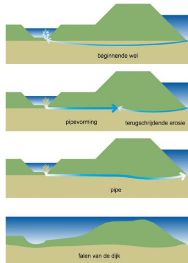
Figuur 3 Schematische weergave piping
