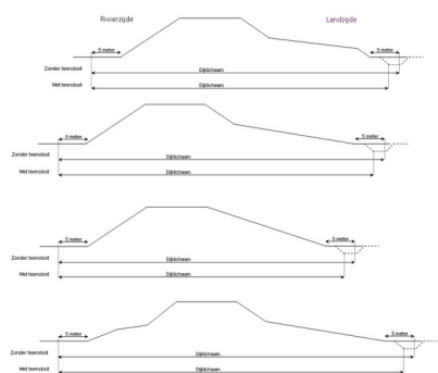
Figuur 3.1 Dijklichaam
