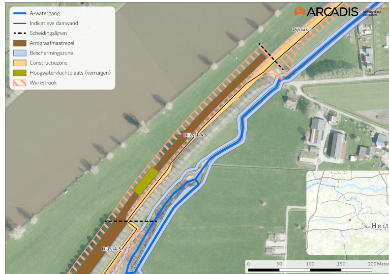
Dijkverbetering Doeveren met (beschermingszone) A-watergang dijkvak 4
