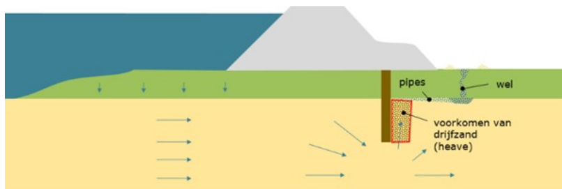
Figuur 4 Werkend principe van een heavescherm
