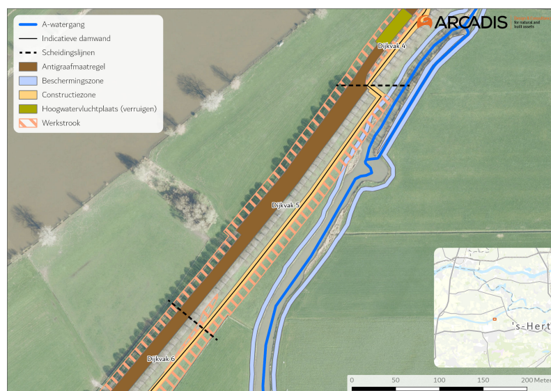
Dijkverbetering Doeveren met (beschermingszone) A-watergang dijkvak 5
