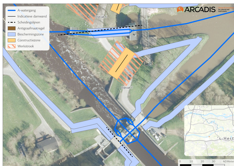
Dijkverbetering Doeveren met (beschermingszone) A-watergang dijkvak 7
