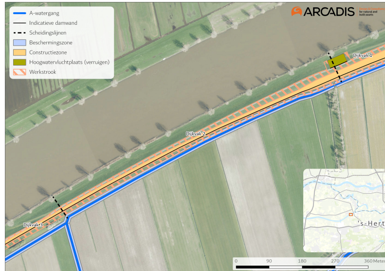
Dijkverbetering Doeveren met (beschermingszone) A-watergang dijkvak 2
