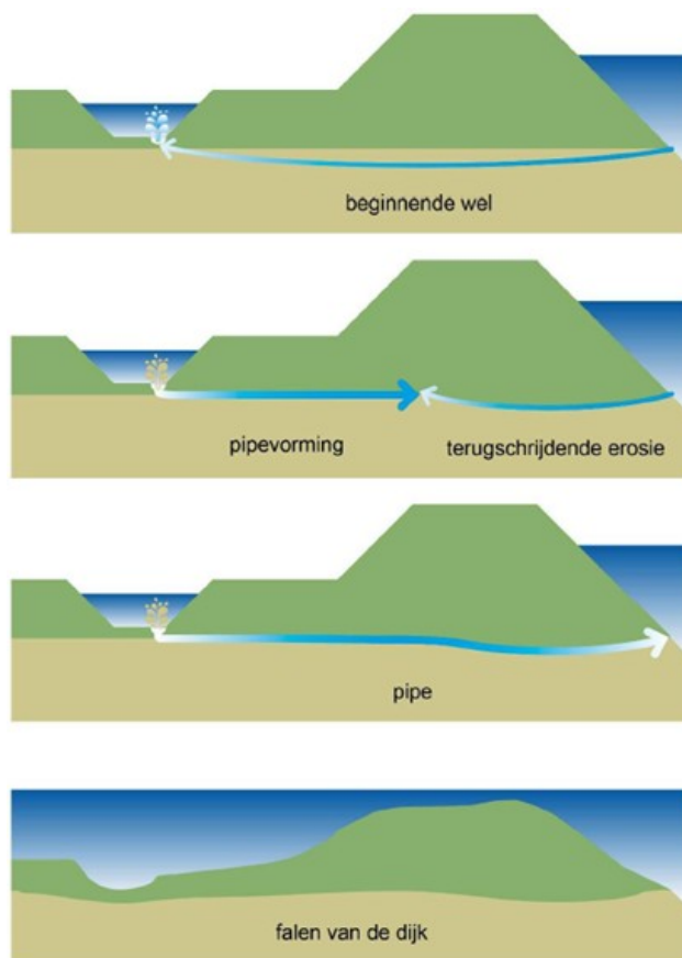
Figuur 3 Schematische weergave piping
