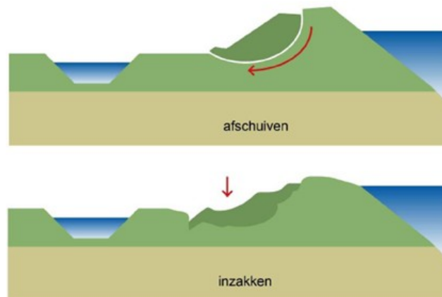
Figuur 2 Schematische weergave macrostabiliteit binnenwaarts
