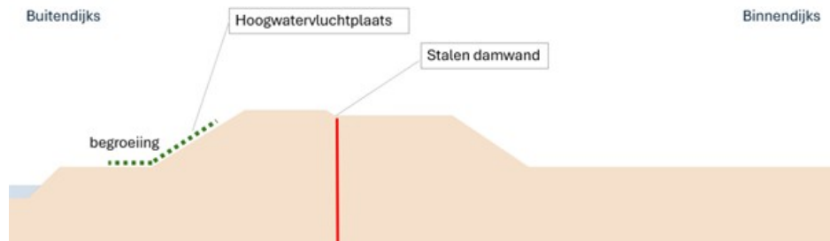
Figuur 16 Schematische weergave van de bevervluchtplaats
