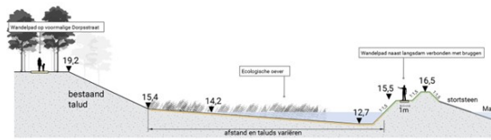
Figuur 4.13 Principe dwarsdoorsnede kom
