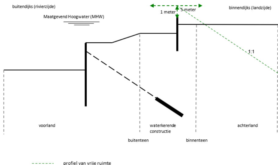
Figuur 2. waterkerende constructie met profiel van vrije ruimte
