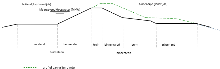
Figuur 1. waterkering met profiel van vrije ruimte
