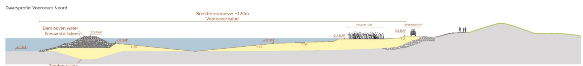
Figuur 3-1: Dwarsdoorsnede van het referentie ontwerp op het traject Meerdijk Noord
