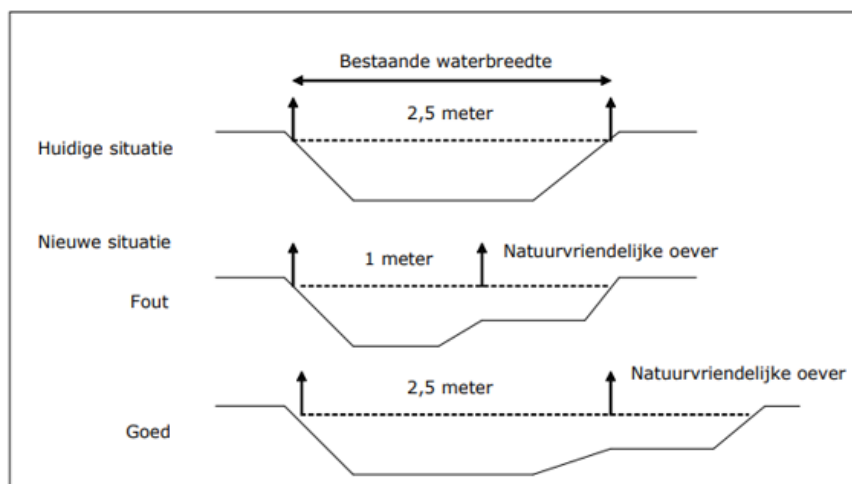
Figuur 1. Voorbeeldtekening van de aanleg van een NVO in een bestaand water. Voor de watergang in dit voorbeeld is het bestaande doorstroomprofiel nodig voor de afvoer. Dat betekent dat de NVO niet binnen de bestaande watergang past, maar dat de watergang verbreed moet worden voor de aanleg van de NVO. Zo verslechtert de doorstroming niet in de nieuwe situatie.
