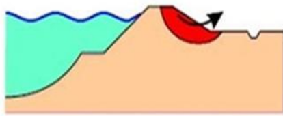
Figuur 2 Schematisch voorbeeld van onvoldoende binnenwaartse stabiliteit
