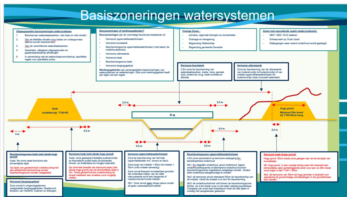
figuur 2.1 schematische weergave van de kernzone en beschermingszone van een watergang en kade
