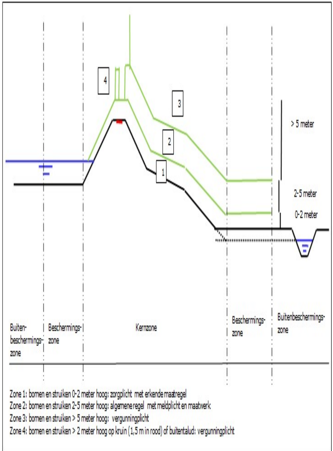
AFBEELDING 23.1 ZONERING VOOR NIEUWE BEPLANTING OP WATERKERINGEN
