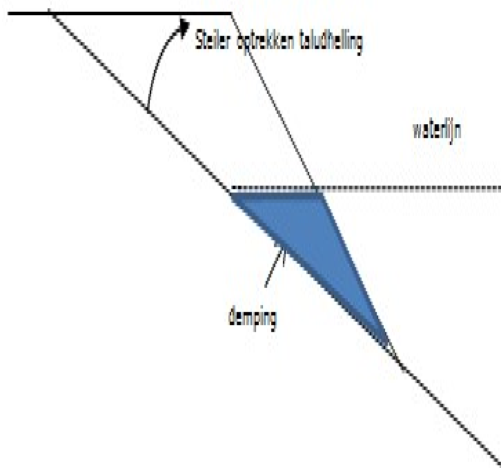
AFBEELDING 3.2 STEILER OPTREKKEN VAN HET TALUD; DEMPING
