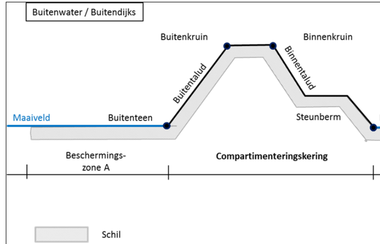
Figuur 25A.1: ligging schil compartimenteringskering
