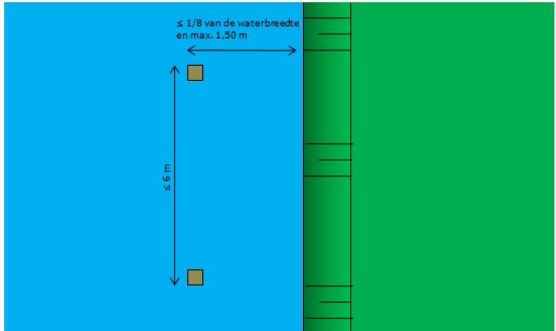
Bovenaanzicht afmeerpaal in water
