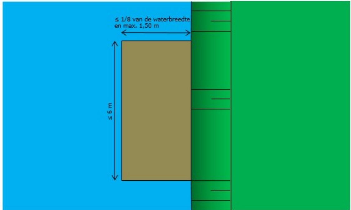
Bovenaanzicht steiger in water (geen waterkering)
