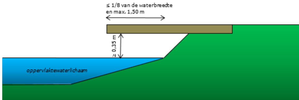
Zijaanzicht vlonder in water (geen waterkering)
