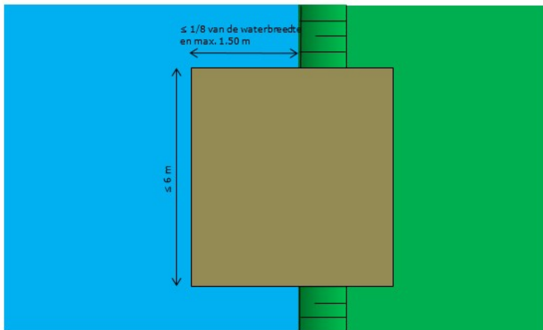
Bovenaanzicht vlonder in water (geen waterkering)
