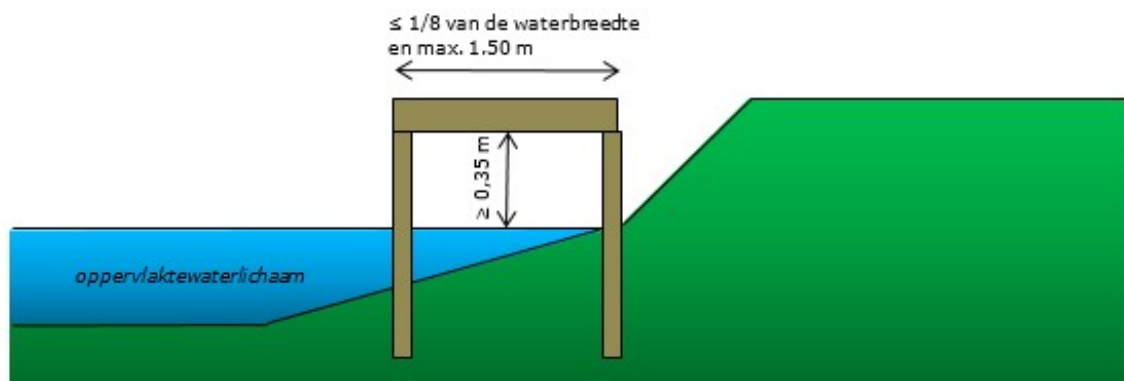
Zijaanzicht steiger in water (geen waterkering)
