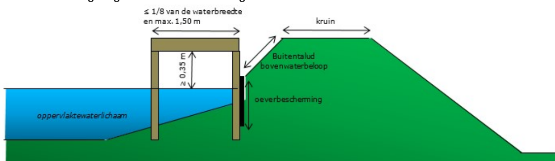
Zijaanzicht steiger in waterkering
