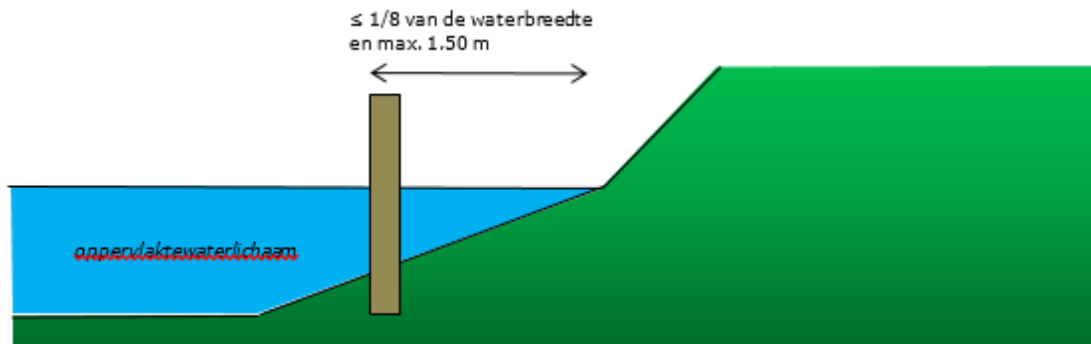
Zijaanzicht afmeerpaal in water
