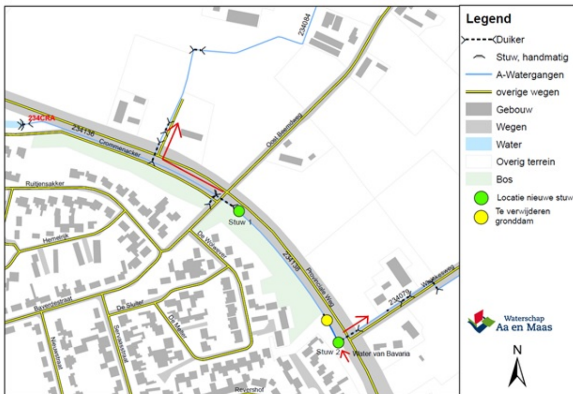
Figuur 1. overzichtskartaal waterverdeling proceswater Bavaria
