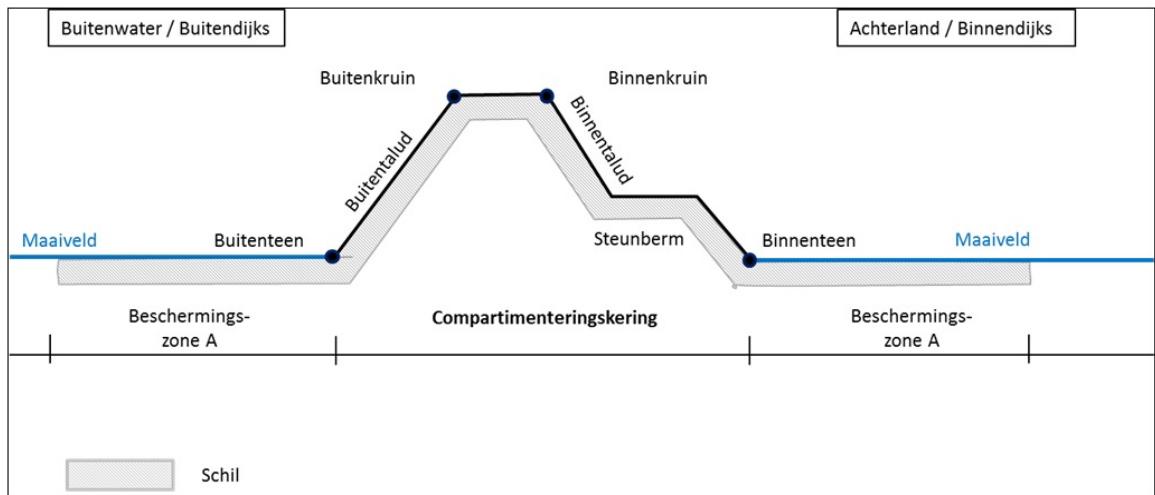
Figuur 25A.1: ligging schil compartimenteringskering
