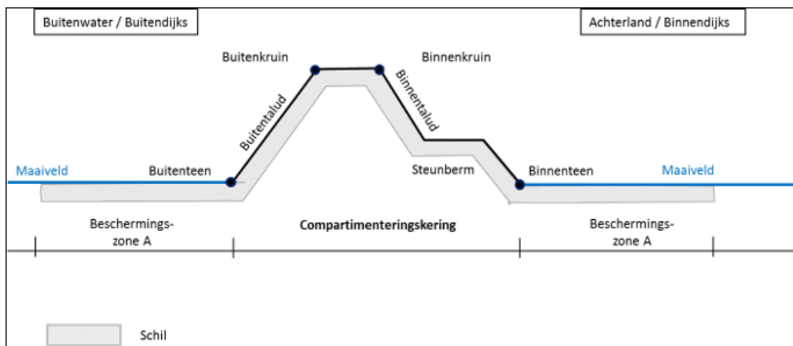
Figuur 25A.1: ligging schil compartimeteringskering
