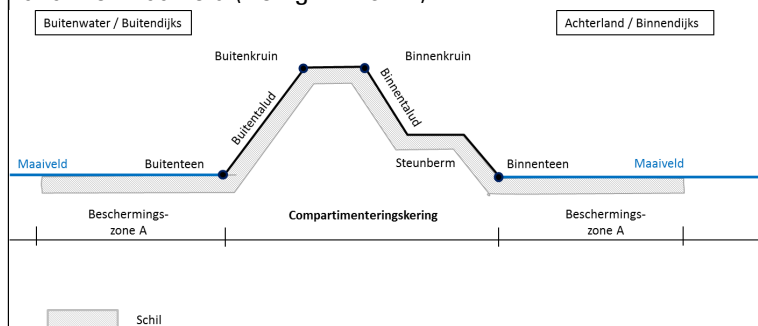
Figuur 25A.1: ligging schil compartimenteringskering
