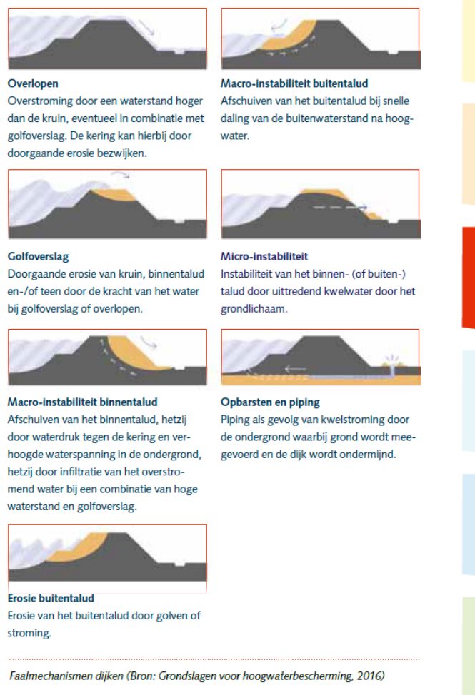
Figuur 15.1: Faalmechanismen waterkeringen (bron: ENW, Grondslagen Hoogwaterbescherming, december 2016)
