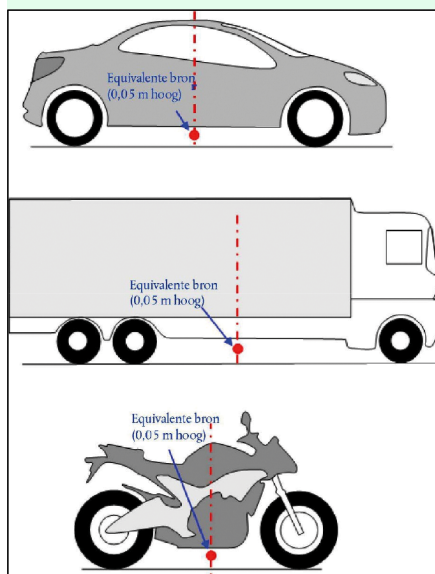
Figuur 2.2.a. Locatie van equivalente puntbron op lichte voertuigen (categorie 1), zware voertuigen (categorieën 2 en 3) en tweewielers (categorie 4)
