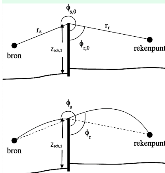
Figuur 4.10: Straalkromming
