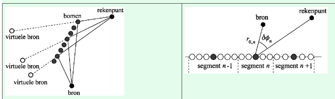
Figuur 4.18a: De bijdrage van een cilinder aan een diffuse reflectie wordt gerepresenteerd door een virtuele bron. Een virtuele bron ligt in het verlengde van de lijn van de cilinder naar het rekenpunt. De afstand van de virtuele bron naar de cilinder is gelijk aan de afstand van de echte bron naar de cilinder.
