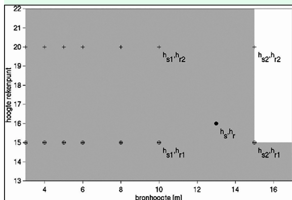
Figuur 4.2b: Detail van figuur 4.2a. Aangegeven is hoe de geluidoverdracht door interpolatie kan worden bepaald.
