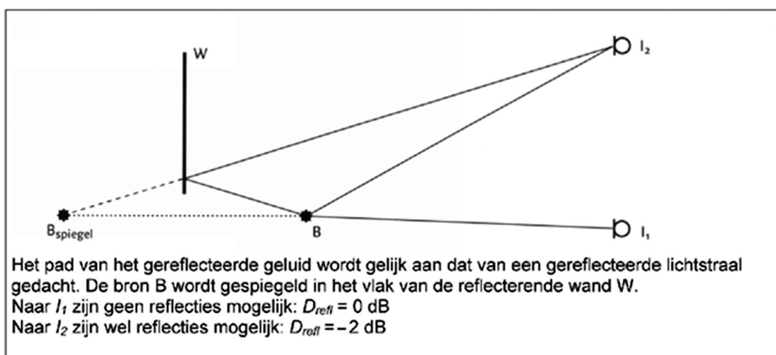
figuur Figuur 2.1 Toelichting op optische spiegeling
