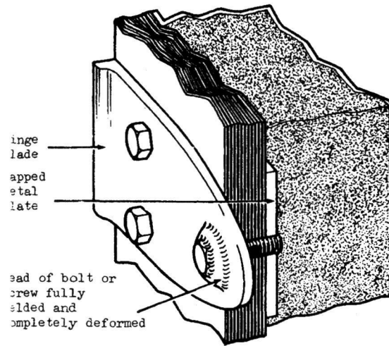
Hinge
