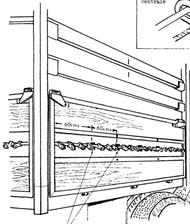
Points de fixation de la barre
