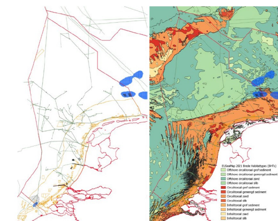
Figuur 7.2. Nederlandse deel van de Noordzee met links een overzicht van alle structuren (windturbines, platforms, leidingen en zandwingebieden zowel actief als verlaten) die potentieel leiden tot verlies of aantasting van benthische habitats. Het blauwe raster presenteert gebieden waar in 2021 op basis van modelberekeningen (Zijl & Laan, 2022) de reductie van het temperatuurstratificatieverschil >20% bedraagt ten gevolge van de aanwezigheid van windmolenparken. Rechts dezelfde kaart, maar nu met een ondergrond die de ligging van de brede habitattypen (EUSeaMap 2021: Vasquez et al., 2021) in de Nederlandse Noordzee laat zien.
