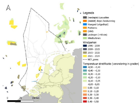
Figuur 7.1. Ruimtelijk beeld van menselijke activiteiten die permanente wijzigingen van de hydrografische eigenschappen in de Nederlandse Noordzee tot gevolg hebben (inclusief de verandering in temperatuurstratificatie op jaarlijkse gemiddelde waarde binnen de Nederlandse Noordzee door de aanleg van windparken). Bij windparken is onderscheid gemaakt in periodes van realisatie. De windparken die in 2022-2024 zijn gepland vallen buiten de huidige beoordeling. De buitenlandse windparken zijn opgenomen vanwege een mogelijke 'externe werking' van synergetische effecten (zie hoofdstuk voor toelichting). Van de pijpleidingen zijn alleen de dikere (> 40 cm) weergegeven, inclusief het deel dat bij de kust is ingegraven.
