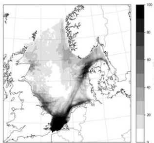
Figuur 11.6. Dominantiekaart voor een LOBE van 20 dB van het Excess Level. LOBE staat voor het 'Level of Onset of Biological Adverse Effects' en is het geluidsniveau waarop dieren ander gedrag beginnen te vertonen (bijvoorbeeld vermijding).
