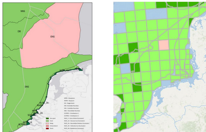
Figuur 5.8. Beoordeling zuurstofcondities in het Nederlandse deel van de Noordzee over de periode 2015-2020, per deelgebied (links) en op basis van 60x60 km gridcellen (rechts). Bron: figuur rechts .
