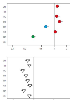
Figuur 8.2. Metaalconcentraties in het sediment van de Zuidelijke Noordzee. Boven: relatieve afstand tot de milieunorm (grijze streep). De gemiddelde concentratie is significant ( p < 0,05 ) hoger (rood) of lager (blauw) dan de milieunorm, of lager dan de achtergrondwaarde (groen). Onder: Trends (jaarlijkse percentage verandering) ten opzichte van de grijze lijn. Driehoek met punt naar beneden: de gemiddelde concentratie neemt significant af ( p < 0,05 ). Ook het 95 procent-betrouwbaarheidsinterval is weergegeven (horizontaal).
