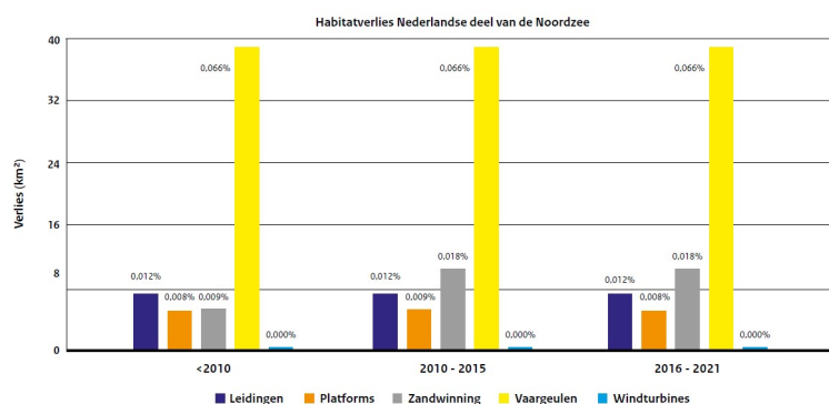
Figuur 6.2. Berekend habitatverlies in het Nederlandse deel van de Noordzee (km² en %) in verschillende periodes volgens de aanvullende nationale analyse.
