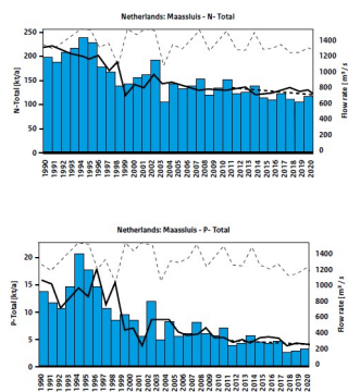
Figuur 5.3. Vrachten van totaal stikstof (boven) en totaal fosfor (onder) van de Rijn bij Maasvluis (in kiloton/jaar). De staven geven de gemeten vrachten aan; de zwarte getrokken lijn de genormaliseerde vrachten, die worden gecorrigeerd voor het gemiddelde debiet per jaar van de rivier. De onderbroken zwarte lijn geeft de trend in genormaliseerde vrachten over de periode 2010-2020. De lichte stippe lijn en de rechter verticale as geven het debiet in m³/s.
