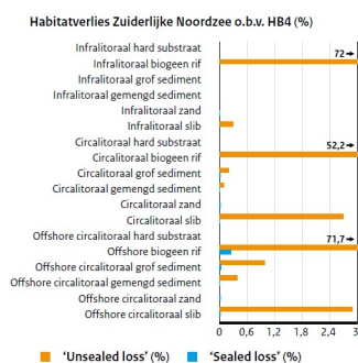
Figuur 6.8. Percentage habitatverlies per breed habitat-type (BHT) in de Zuidelijke Noordzee op basis van de OSPAR BH4-beoordeling (Schmitt et al., 2023) met onderscheid in 'sealed loss' (verlies door leidingen, platforms en windmolens) en 'unsealed loss' (verlies door bodemberoerende activiteiten).
