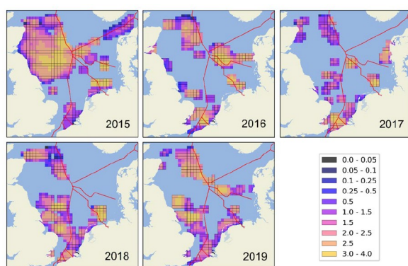
Figuur 11.3. Jaarlijkse risicokaarten voor de periode 2015 tot en met 2019 voor de bruinvissen, zoals die zijn berekend voor de OSPAR-beoordeling van het risico van impact van impulsgekluid. De weergave heeft een logaritmische schaal. Per gridcel is de logaritme (basis 10) weergegeven van het aantal bruinvisverstoringsdagen gedeeld door het aantal dagen per jaar. Door de herleiding naar daggemiddelden kunnen ook maandelijkse kaarten (waarvoor hetzelfde gebeurt) op dezelfde schaal worden weergegeven.
