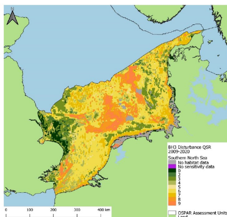
Figuur 6.6. Mate van aantasting van de zeebodem van de Zuidelijke Noordzee over de periode 2009-2020, zoals berekend met de OSPAR BH3-indicator op basis van visserijdrukpatronen (gemiddelde waarden per ICES c-square).
