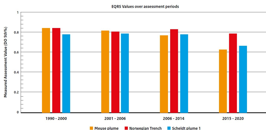
Figuur 5.9. EQRS-waarden gebaseerd op gemeten zuurstofconcentraties (5 procent laagste waarnemingen) verslechteren significant in de Maaspluim en de Scheldepluim 1 in de periode 1990-2020.
