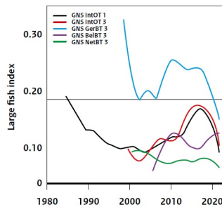
Figuur 4.6. Tijdreeks van de Large Fish Index (LFI) per m 2 eetnet. De drempelwaarde is weergegeven met een zwarte horizontale lijn op y=0.17 , en tijd in jaren op de x-as. De kleuren geven de trends per survey weer. Dit bijschrift verwijst alleen naar de surveys die relevant zijn voor de Nederlandse Mariene Strategie: zwart de Greater North Sea International Otter Trawl, eerste kwartaal (GNSIntOT1) en rood de Greater North Sea International Otter Trawl, derde kwartaal (GNSIntOT3).
