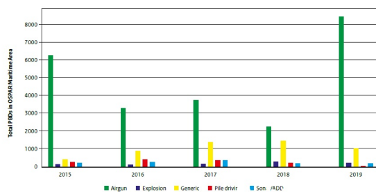
Figuur 11.2a. Pulsblokdagen in de gehele OSPAR-regio in de periode 2015-2019, per geluidsbron.
