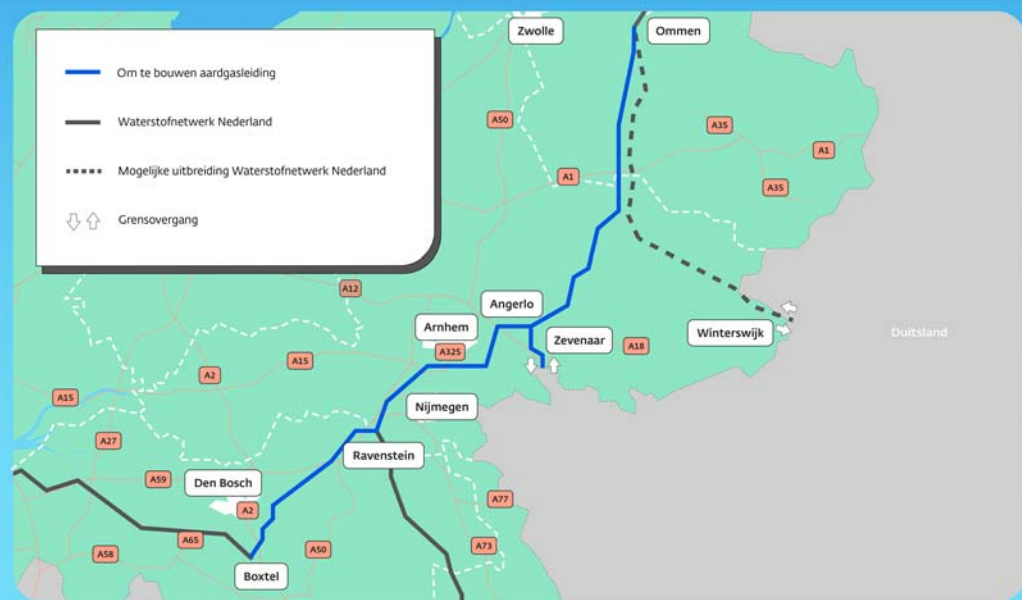
Figuur 1 – Schematische weergave van het Waterstofnetwerk Nederland
