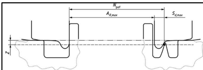
Figuur 5: Leidmaat A_{R,max} + S_{d,max} en strijmaat N_{pof}
