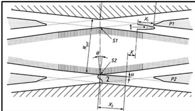
Figuur 6: Bovenaanzicht met N_{\text{perp}} en aanloophoek \alpha
