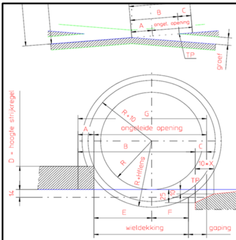
Figuur 4: Overzicht ongeleide opening
