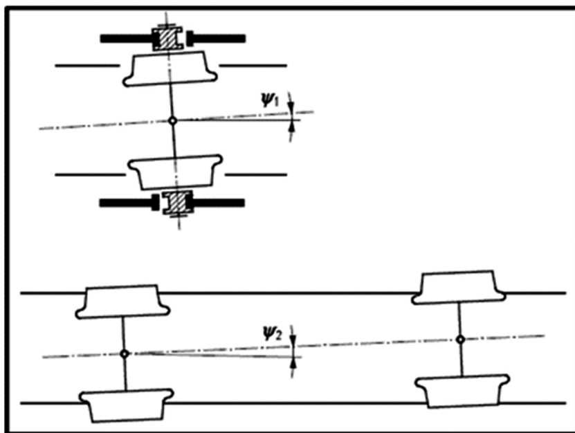
Figuur 3: Overzicht aanloophoeeken
