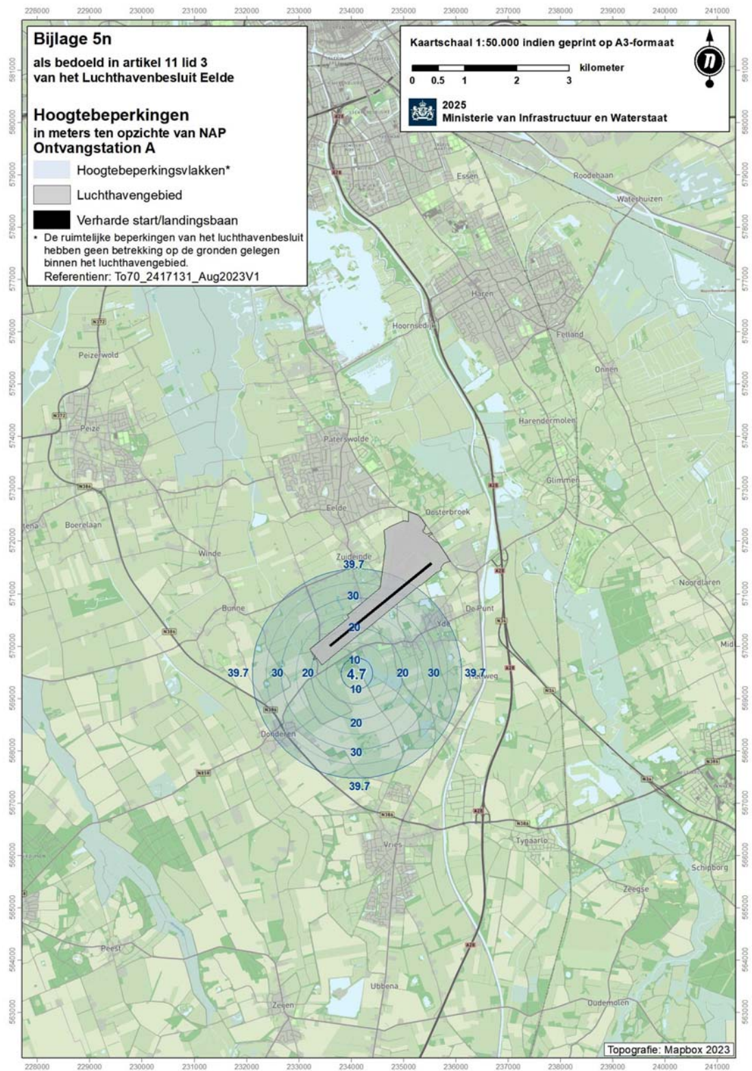
Kaart (1:50.000) met hoogtebeperkingen: Surface voor ontvangststation A
