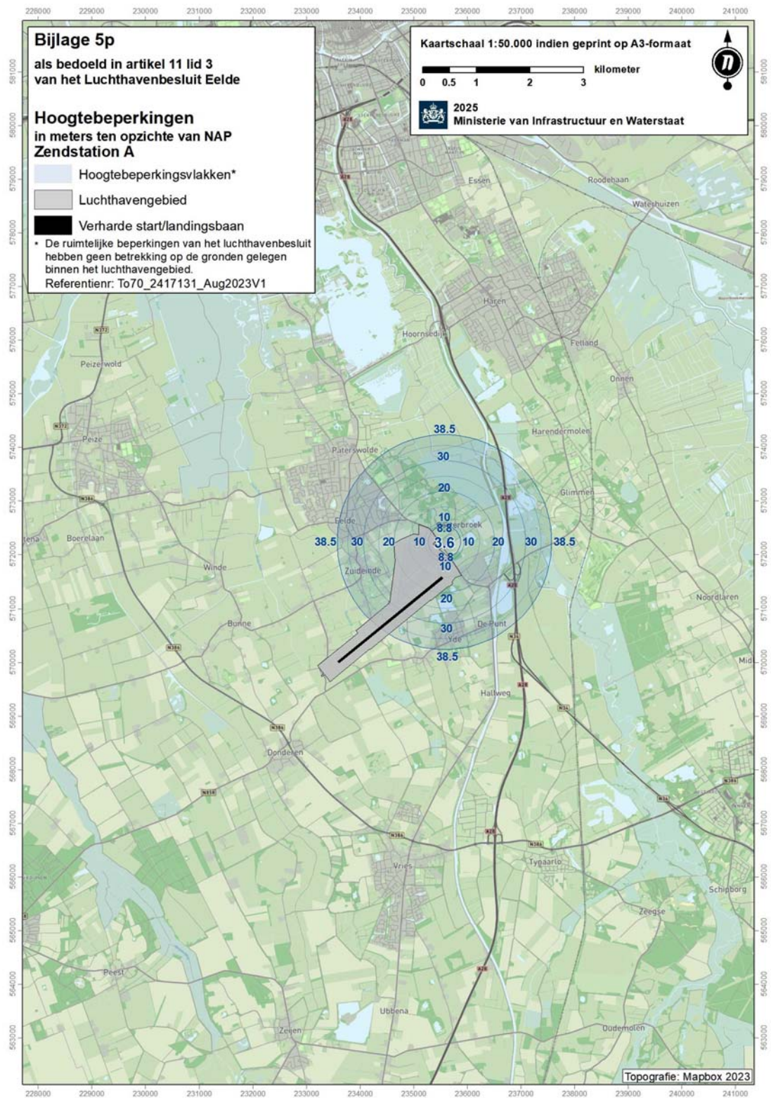
Kaart (1:50.000) met hoogtebeperkingen: Surface voor zendstation A
