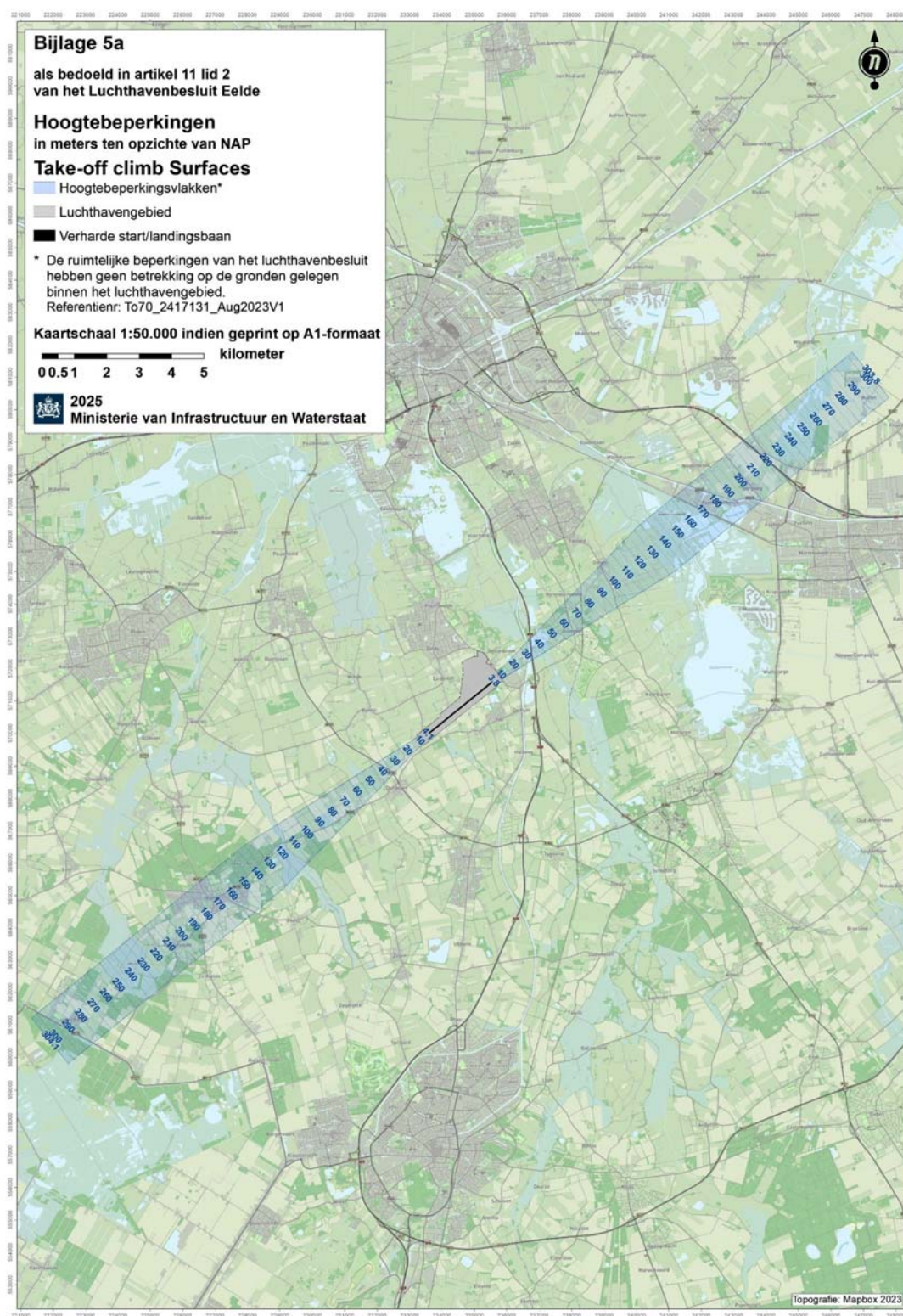
Kaart (1:50.000) met hoogtebeperkingen: Take-off climb Surfaces
