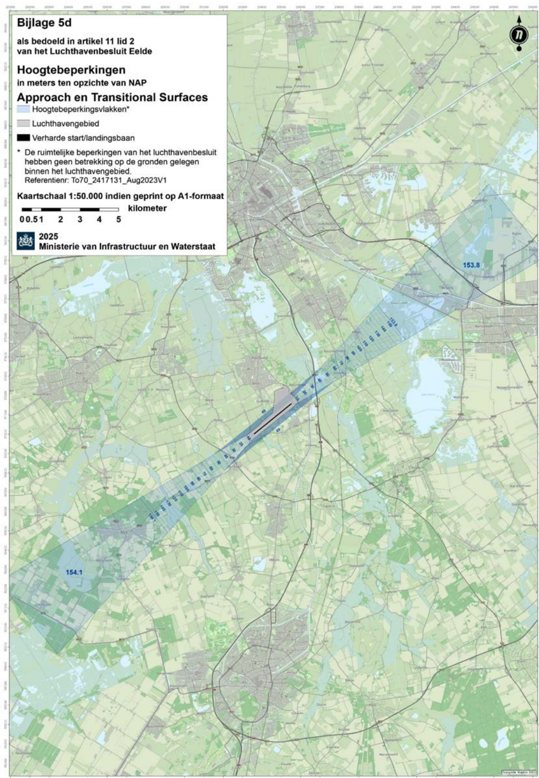
Kaart (1:50.000) met hoogtebeperkingen: Approach en Transitional Surfaces
