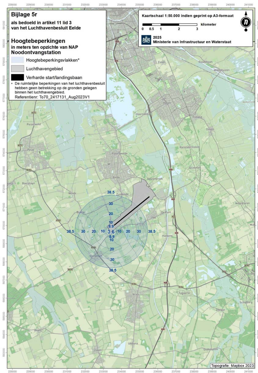
Kaart (1:50.000) met hoogtebeperkingen: Surface voor noodontvangstation
