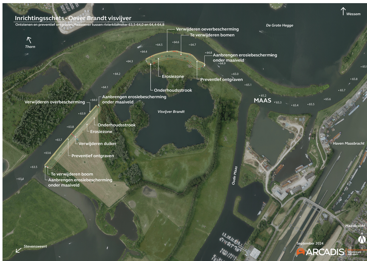
Figuur 10. Inrichtingsschets KRW-maatregel Oever Brandt-Visvijver.
