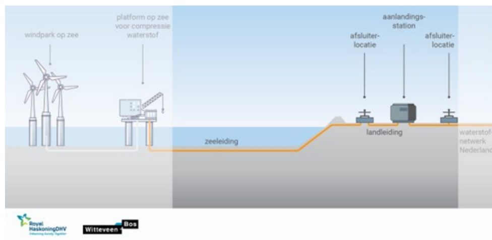
Afbeelding 6: Schematische weergave van een waterstofverbinding
