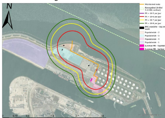
PR-contouren van de zeeleiding op land en microtunnel (exclusief aanvullende mitigerende maatregelen)
