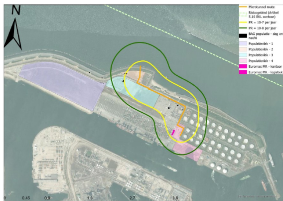
PR-contouren van de zeeleiding op land en microtunnel (inclusief aanvullende mitigerende maatregelen)
