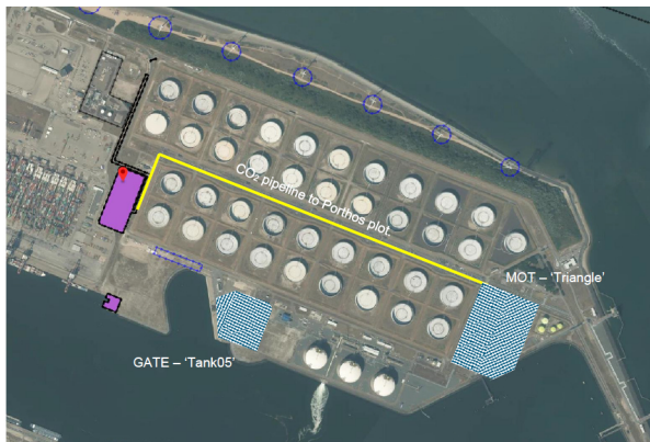
Figuur 4.7 Alternatieven CO2-terminal
