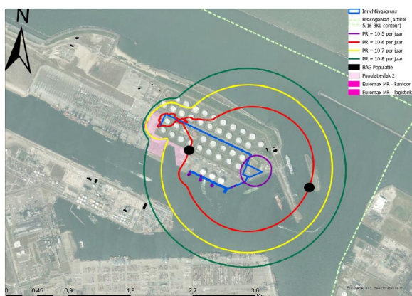
PR-contouren van de CO 2 -terminal
