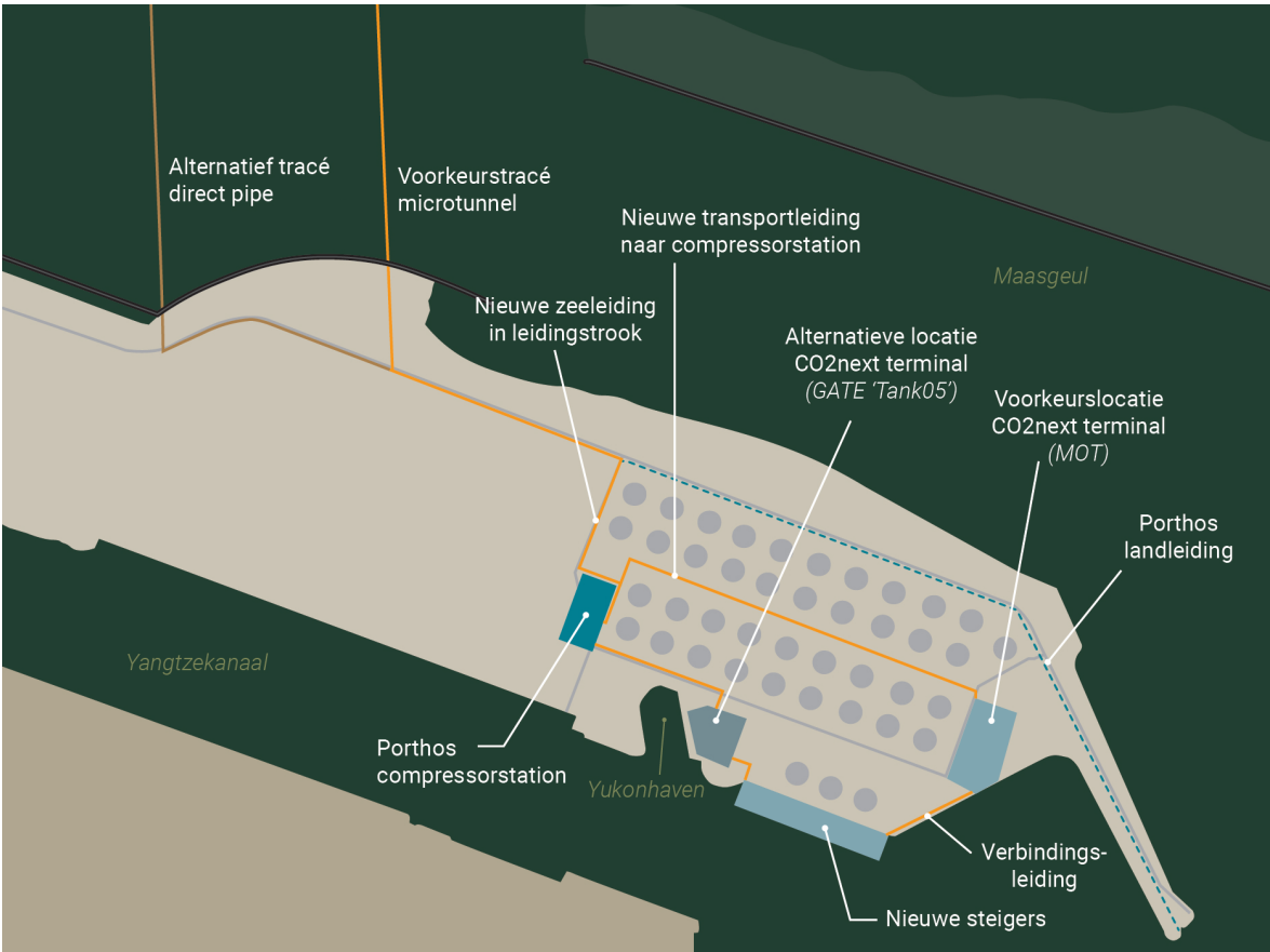
Figuur 4.5 Ruimtelijke alternatieven op land
