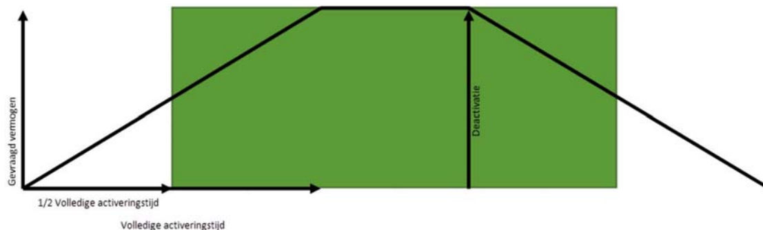
Figuur 1 – Schematische weergave berekening geactiveerd volume noodvermogen per onbalansverrekeningsperiode
