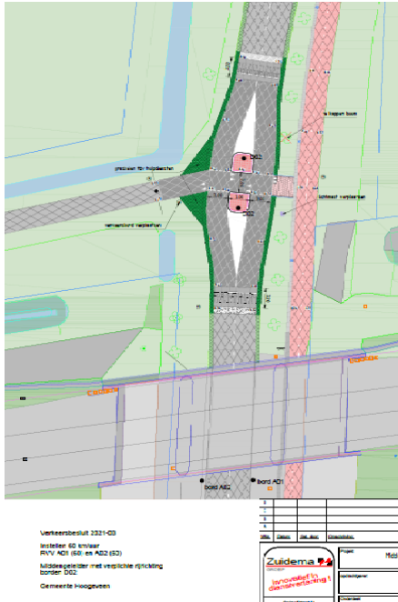
- Situatietekening Zuidwoldigerweg te Hoogeveen
