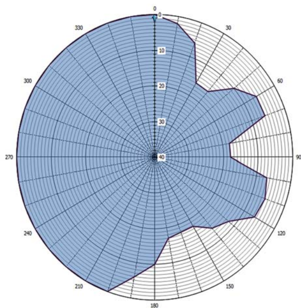
Grafische weergave antennediagram (0 = geografisch Noorden)
