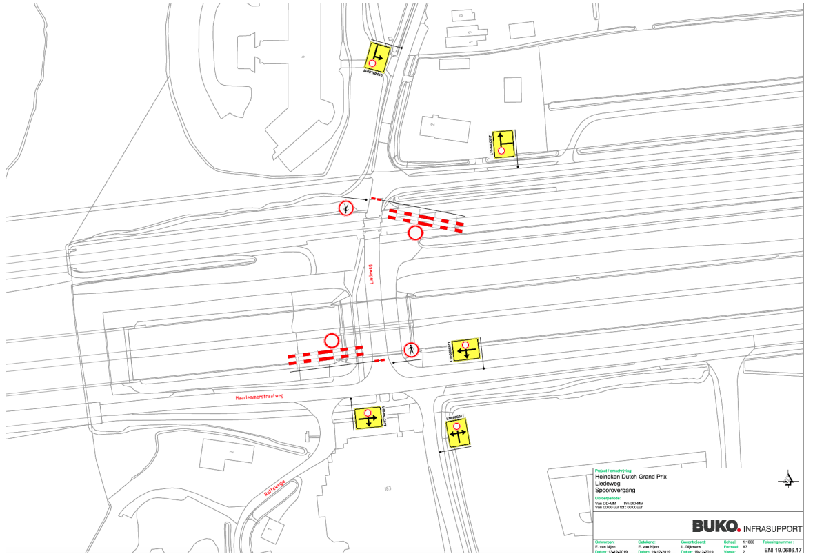
Situatieschets Vinkebrug
