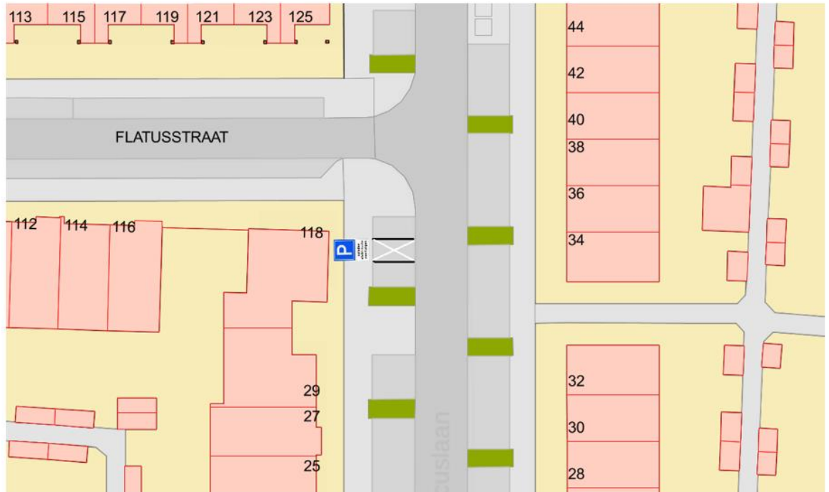
Bebordingstekening 1 o Articusstraat
