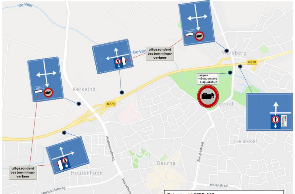
Tekening V-0555-003 Behoort bij Verkeersbesluit 16 april 2019 Verbod voor vrachtverkeer
