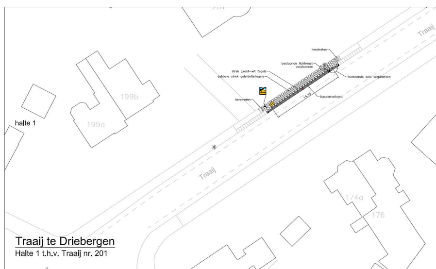
Figuur 2, Schetsontwerp nieuwe halte locatie Traaij-Arnhemsebovenweg
