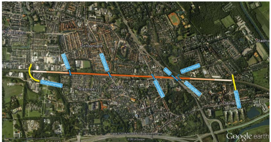
Figuur 2: Verdiepte ligging Vught conform variant V3
