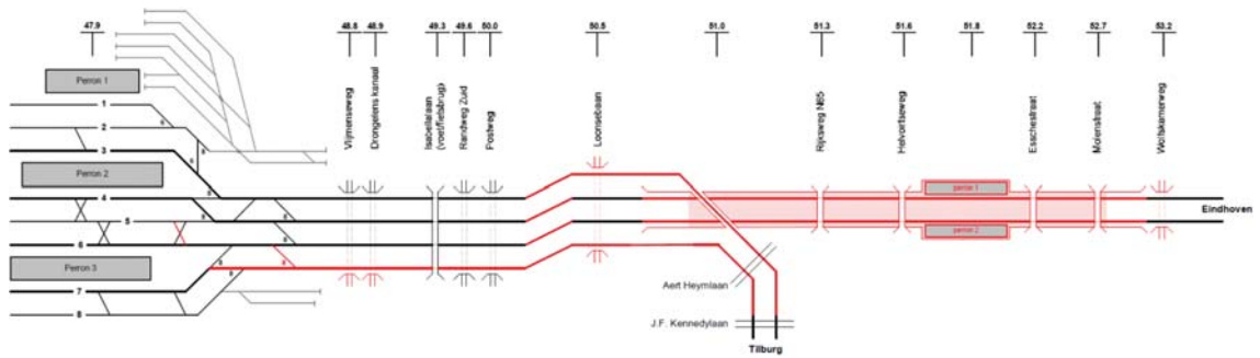
Figuur 2: Verdiepte ligging Vught conform variant V3
