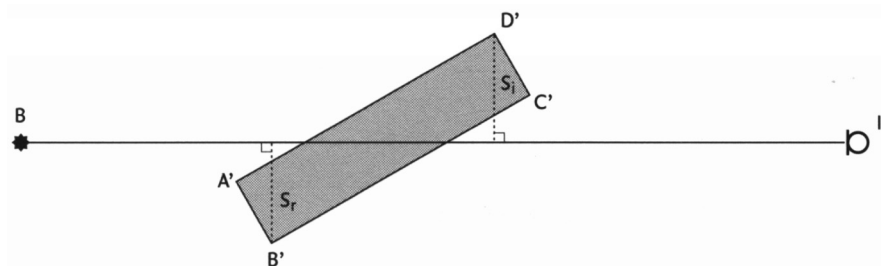
figuur 3.4 Toelichting bij de bepaling van s_i en s_r bij een gebouw
