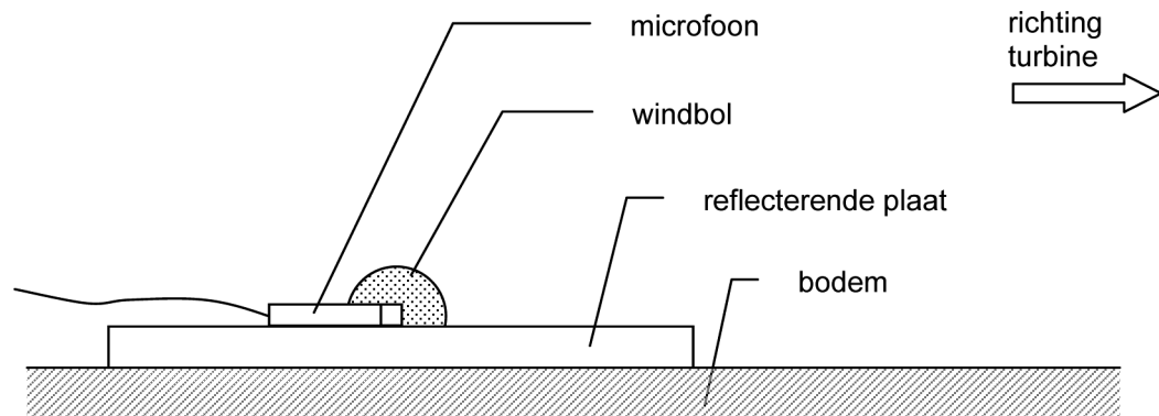
figuur 2.3 weergave van de meetopstelling
