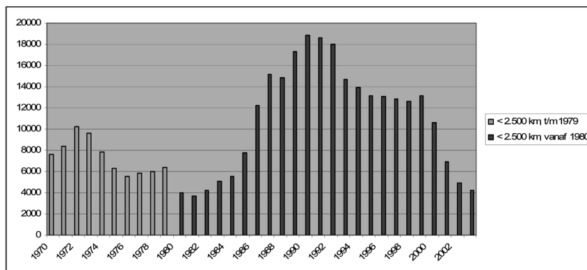
Figuur 6 – aantallen personenauto's naar bouwjaar voor cohort < 2 500 km in 2004
