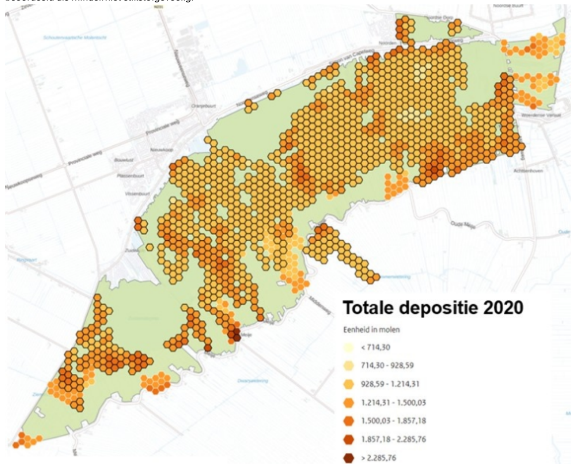
Figuur 8-2. Berekende depositiewaarden in 2020 in Natura 2000-gebied Nieuwkoopse Plassen & De Haeck. De wit omlijnde hexagonen zijn locaties waar H6430A of H6430B ligt. Deze habitattypen hebben een KDW >2400 hebben en door door Wamelink et al., (2023) zijn beoordeeld als minder/niet stikstofgevoelig.
