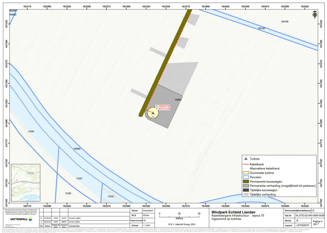
Afbeelding 15 Inrichting windturbine 5
