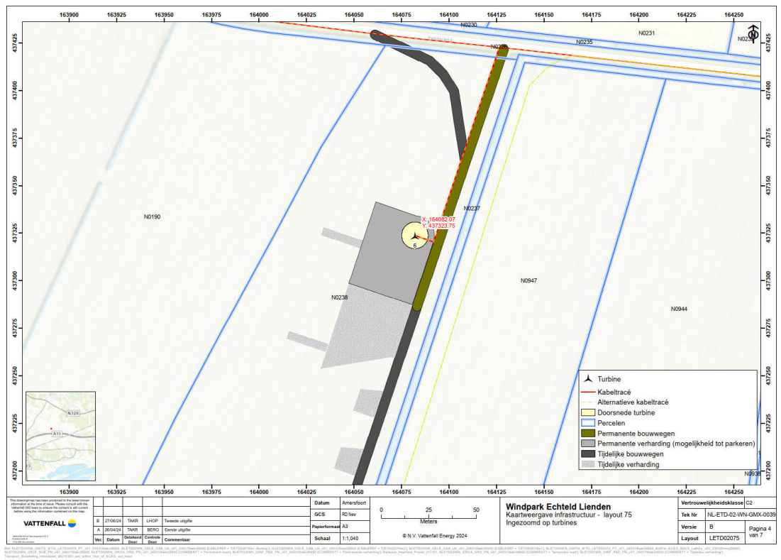
Afbeelding 16 Inrichting windturbine 6
