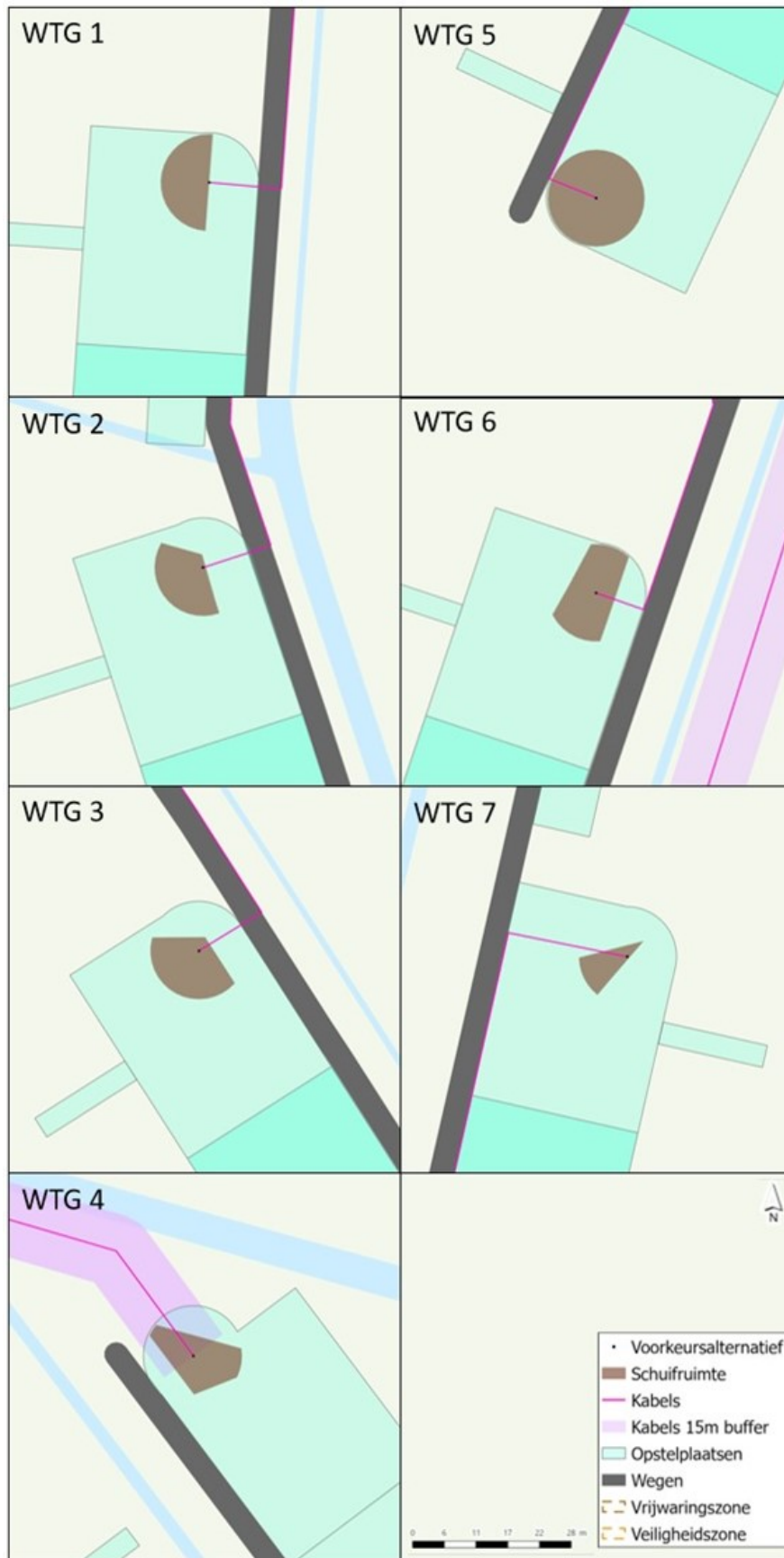
Afbeelding 19: Schuifruimte per windturbine
