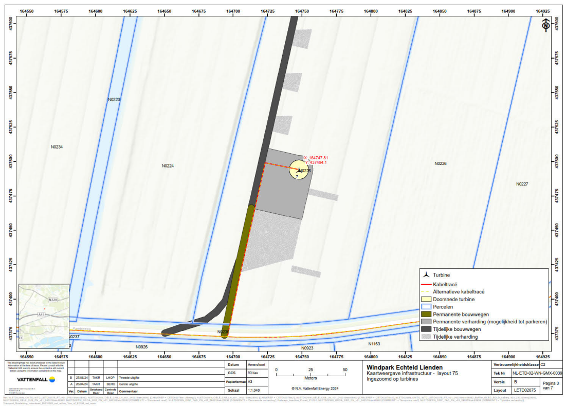
Afbeelding 17 Inrichting windturbine 7
