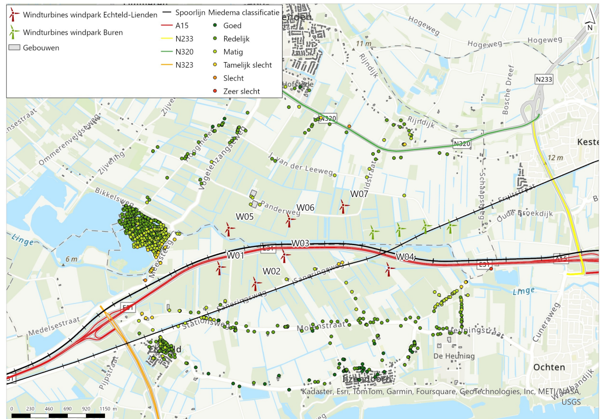
Afbeelding 5.34 Miedema classificatie op de geluidgevoelige gevels van de ondergrens turbines en overige geluidbronsoorten
