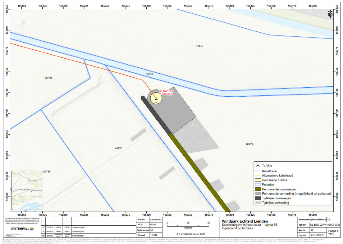
Afbeelding 14 inrichting windturbine 4
