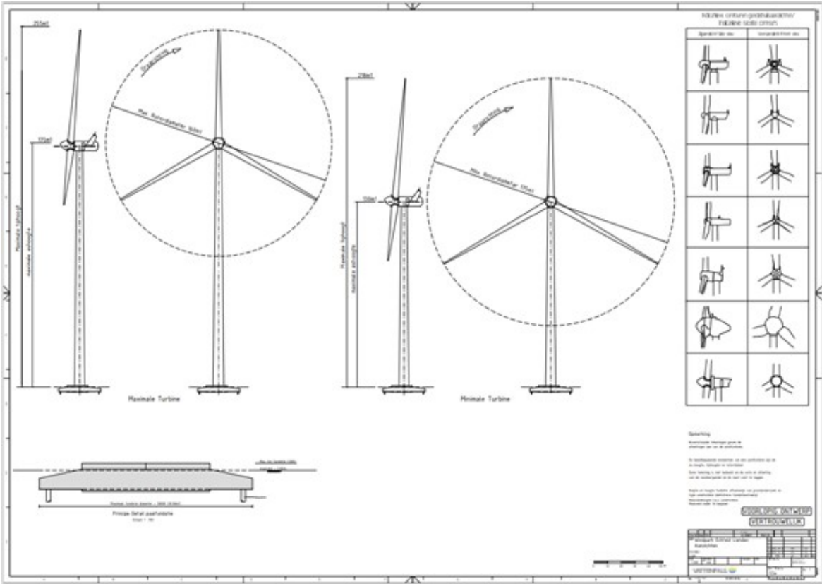
Afbeelding 5 Schematische weergave turbinerange
