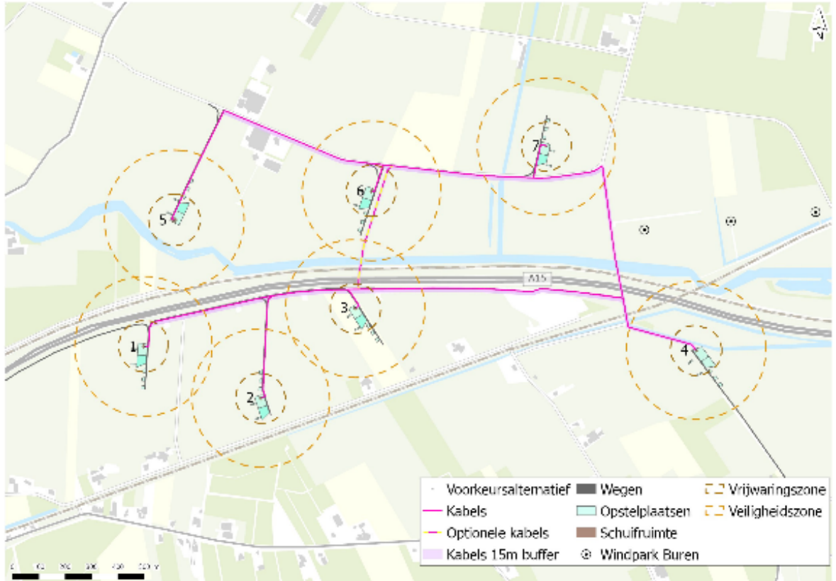
Afbeelding 5.25 Opstelling windturbines
