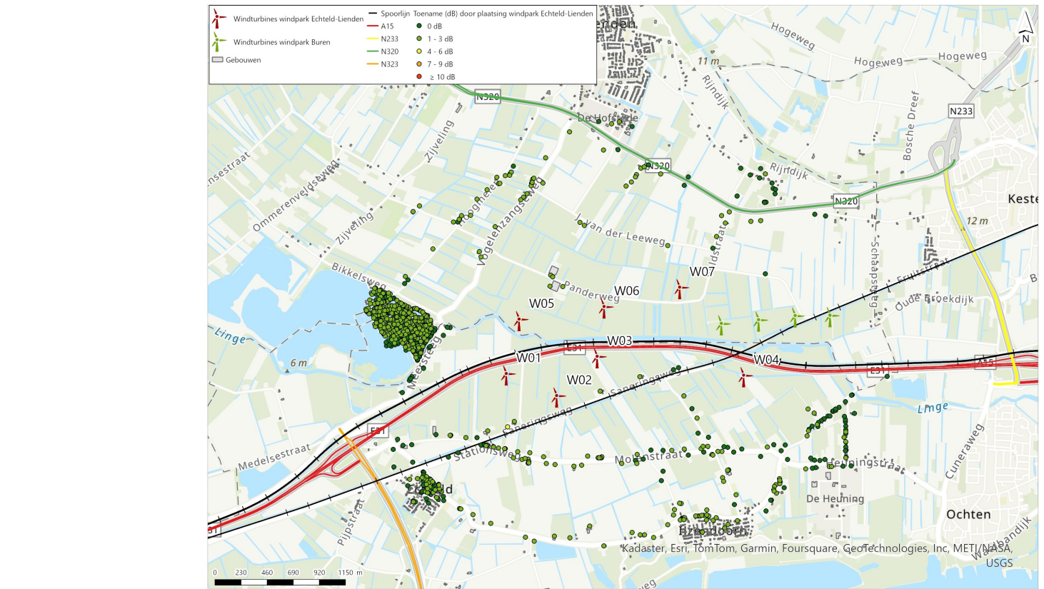
Afbeelding 5.35 Toename van het geluid op de omgeving als gevolg van het plaatsen van de ondergrens turbines van windpark Echteld-Lienden
