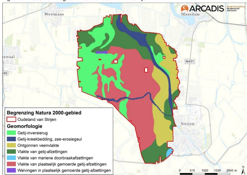
Figuur 5-1: Geomorfologische kaart Oudeland van Strijen.
