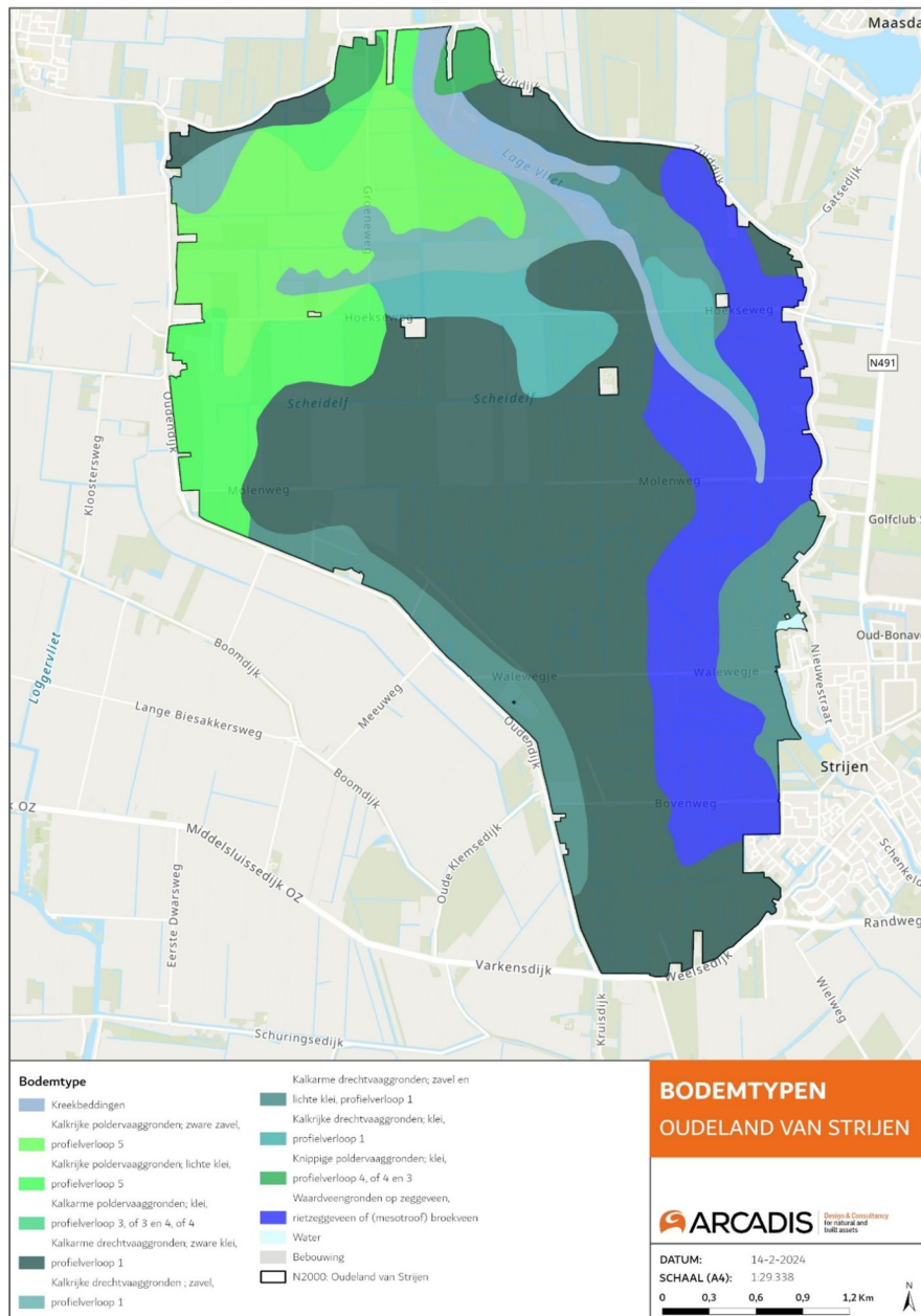
Figuur 5-2: Bodemkaart van het Oudeland van Strijen.
