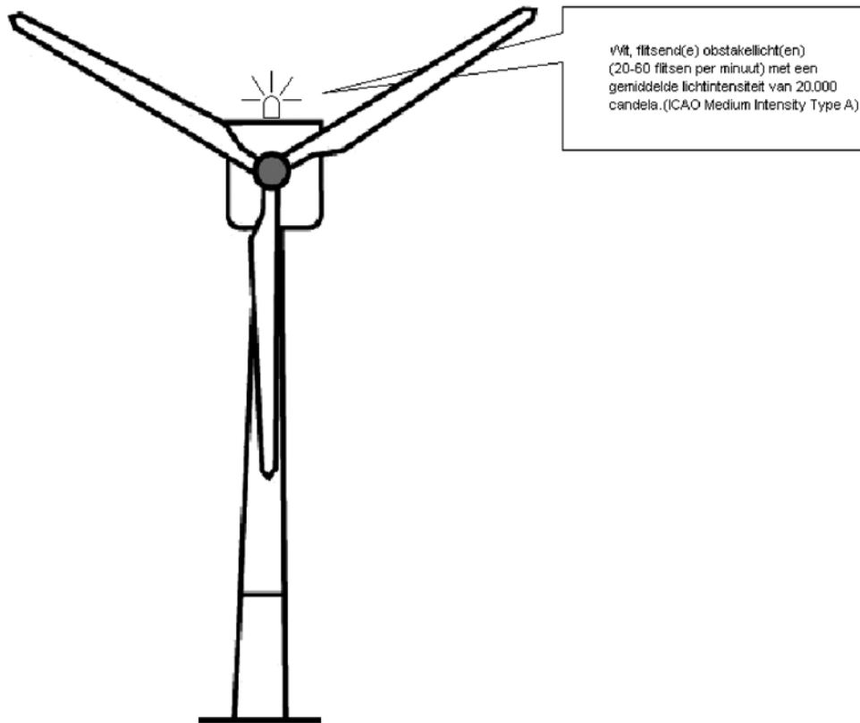
Figuur VI – 1 obstakellichten windturbine tijdens daglichtperiode
