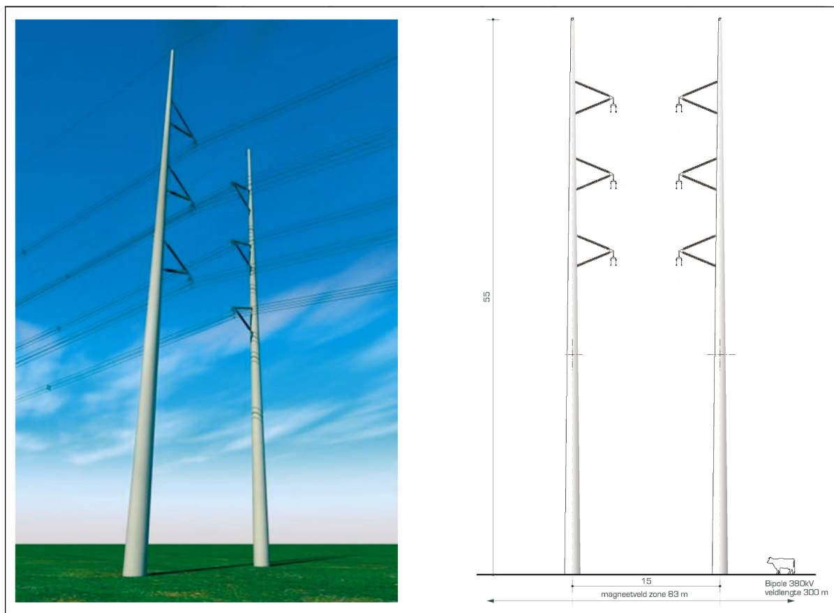
Figuur 1a Impressie voorontwerp M-compactmast (380 kV) 1
