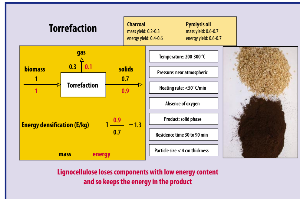
Figuur 8. Torrefactie (bron: presentatie Vergassing en torrefactie, H.J. Veringa, ECN, 2006)
