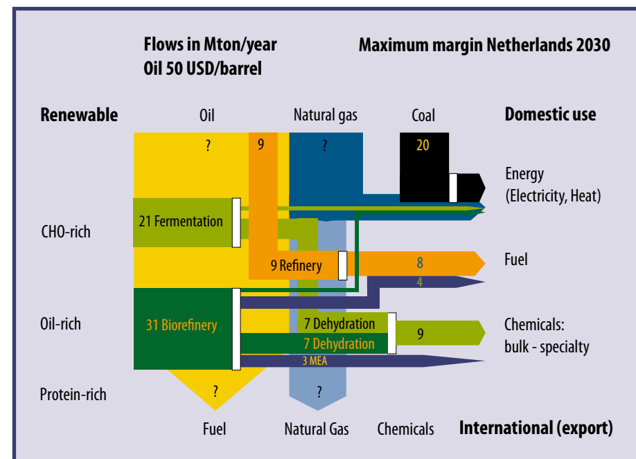
Figuur 18. Energiestromen voor import, binnenlands gebruik en export in Nederland in 2030 (doelstelling 'maximale opbrengst') (bron: Potential of coproduction of energy, fuels and chemicals from biobased renewable resources, WISEBIOMAS, 2006)
