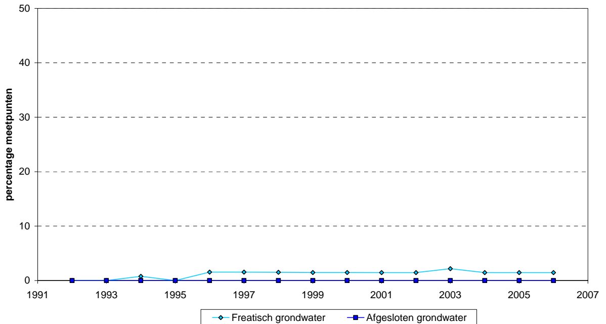
Figuur 28: Overschrijding van de EU-streefwaarde van 50 mg/l voor de gemiddelde nitraatconcentratie in het grondwater op drinkwaterproductielocaties voor freatisch grondwater en afgesloten grondwater in de periode 1992-2002. Overschrijding is weergegeven als het percentage van alle productielocaties.
