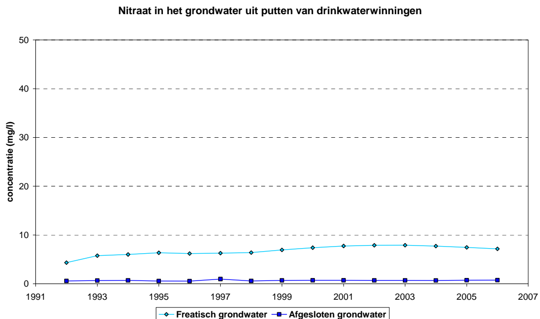
Figuur 27: Gemiddelde jaarlijkse nitraatconcentratie (mg/l) in het grondwater op drinkwaterproductielocaties in freatisch en afgesloten watervoerende pakketten in de periode 1999-2006.
