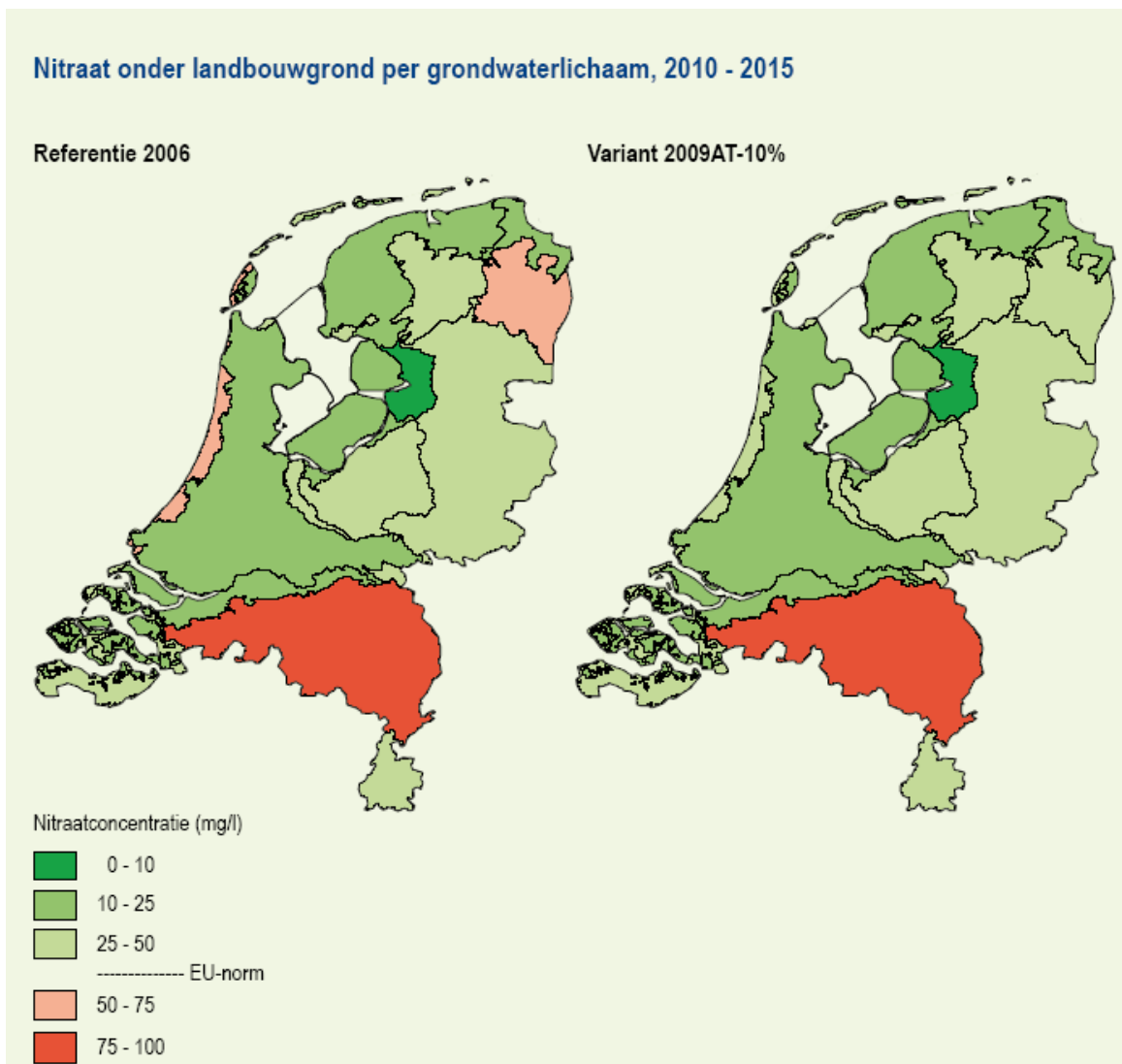
Figuur 44: Schatting van de nitraatconcentratie in 2010-2015 in landbouwgebieden voor de verschillende grondwaterlichamen. Bron: MNP, 2007
