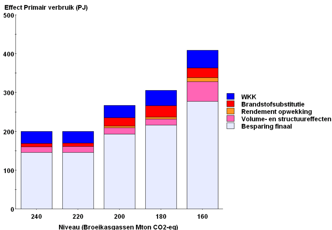
Figuur 5.15 Besparingen, volume- en structureffecten en brandstofsubstitutie bij afnemende BKG-emissies in 2020, ten opzichte van het hoge-olieprijsscenario GE^{ho}
