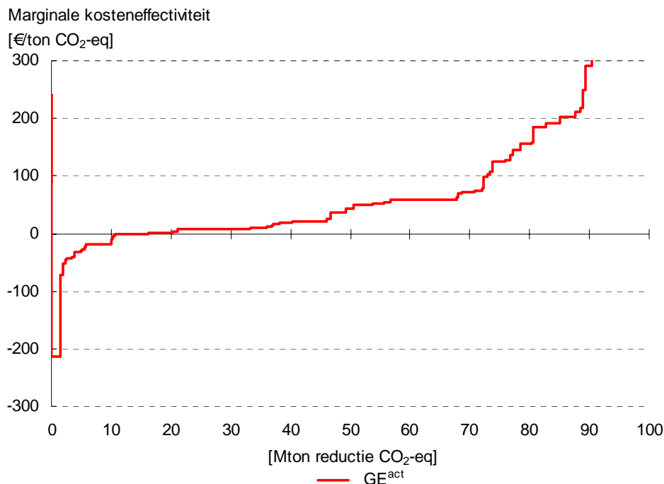
Figuur 5.5 Kostencurve emissiereductie broeikasgassen van 90 Mton CO 2 -eq
