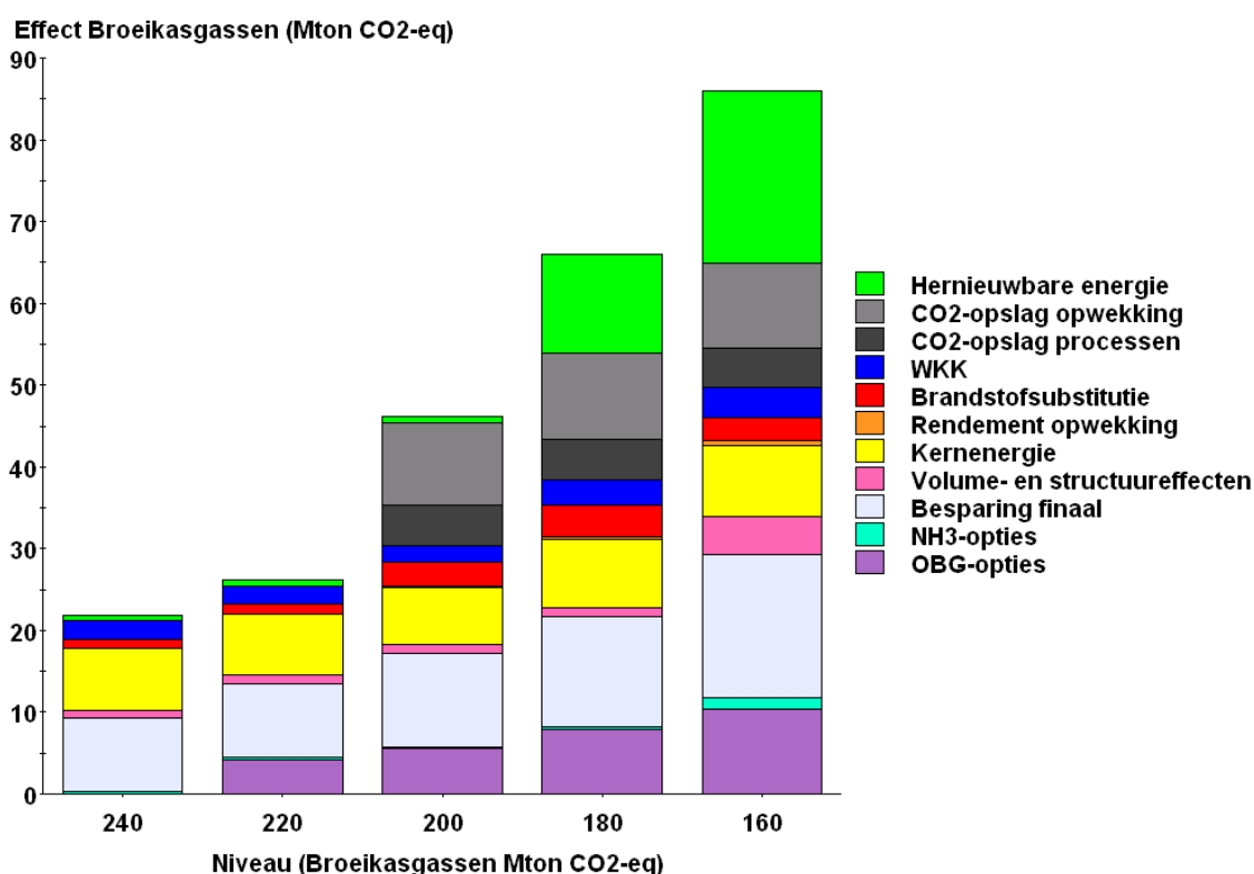
Figuur 5.13 BKG-emissiereducties per categorie in de optiepakketten voor het hoge olieprijs-achtergrondscenario ( GE^{ho} )
