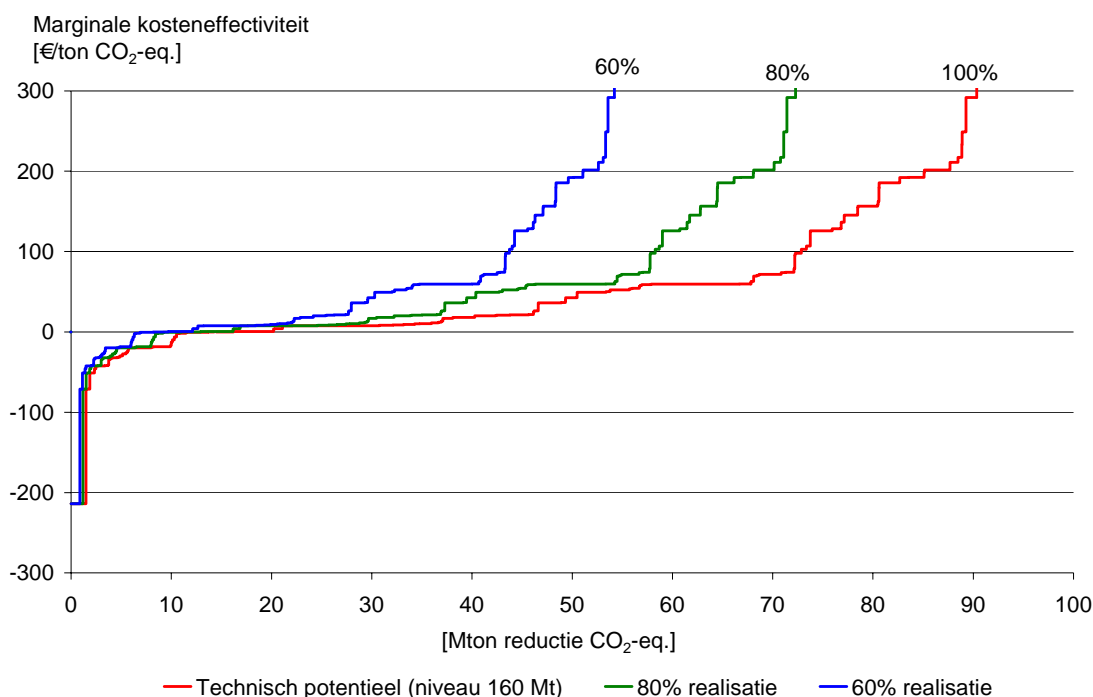
Figuur 6.3 Voorbeeld kostencurves voor technisch potentieel en situaties waarin het realiseerbaar potentieel resp. 60 en 80% van het technisch potentieel is (uitval evenredig verdeeld over alle opties).
