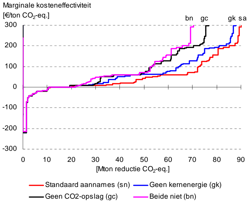
Figuur 5.11 Kostencurves in GE^{act} met en zonder uitsluiting van de opties CO_2 -opslag en kernenergie
