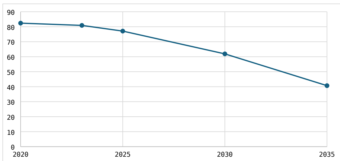
Figuur 3. Stikstofdepositie door wegverkeer op stikstofgevoelige natuur in Natura 2000-gebieden (mol/ha/jaar) 1
