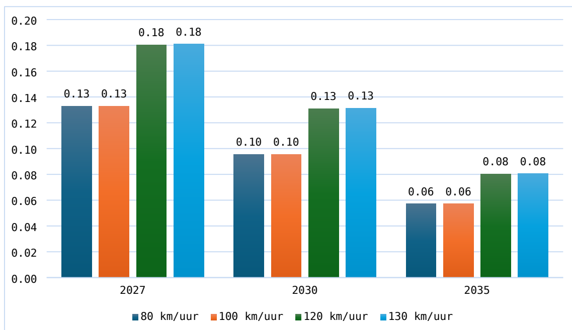
Figuur 5. Gemiddelde NO x -emissie door personenauto's, bestelauto's en motoren op snelwegen (gram/voertuigkilometer) 7
