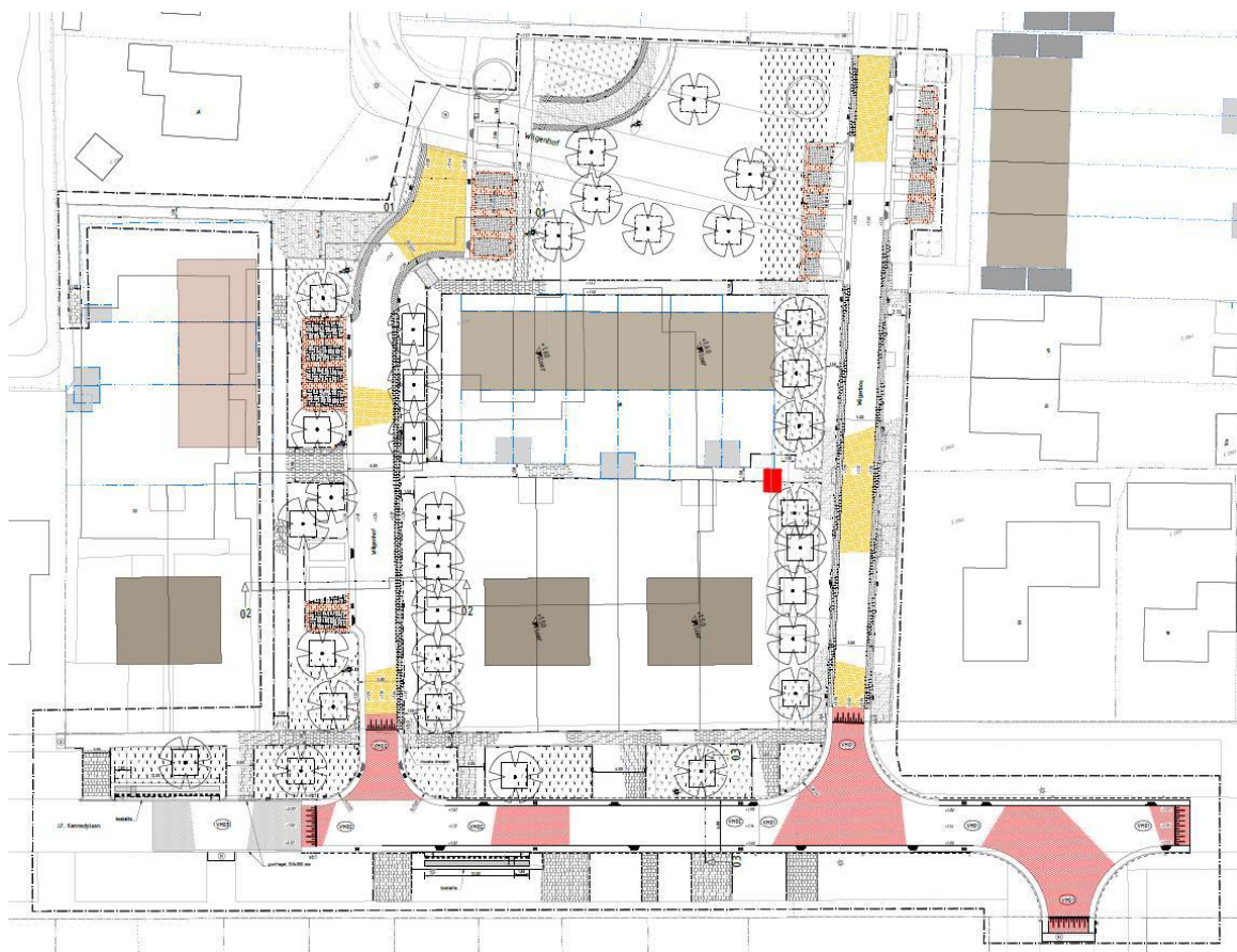
Situatie J.F. kennedylaan/Wilgenhof/Wilgenbos
